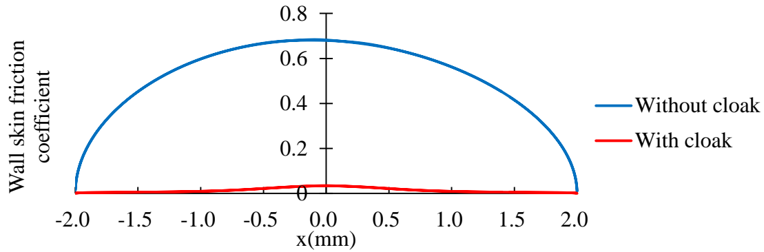
(b) Re=15
