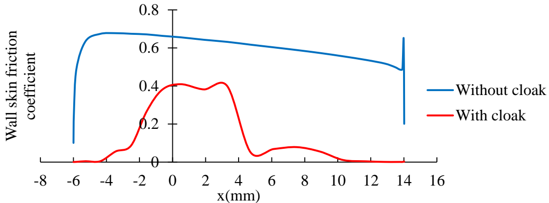
(b) Re=10
