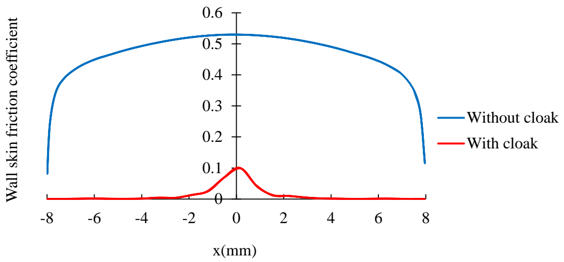
(b) Re=15
