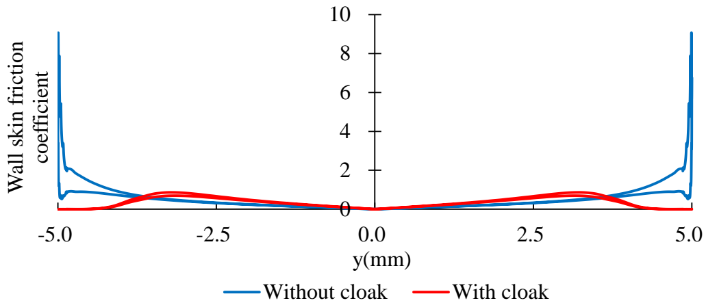
(b) Re=10
