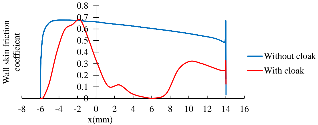
(b) \text{Re}=10
