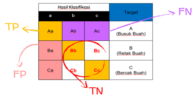
Gambar 6. Ilustrasi perhitungan menggunakan teknik ROC
