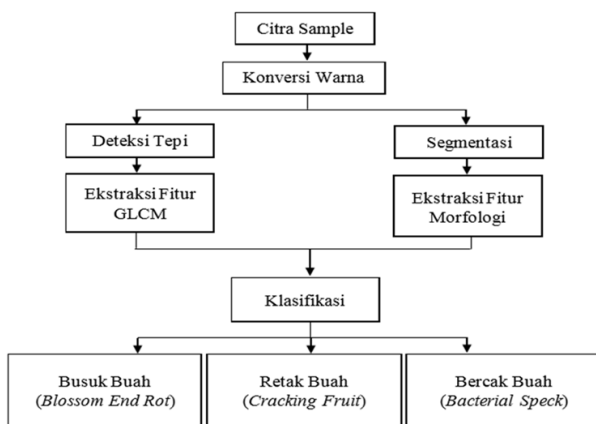
Gambar 1. Diagram blok klasifikasi kerusakan mutu tanaman tomat
