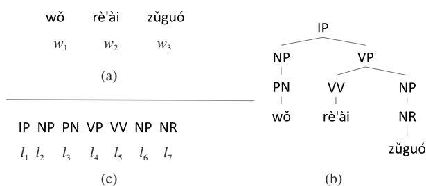
图 7 源端句子“我热爱祖国”的词序列
