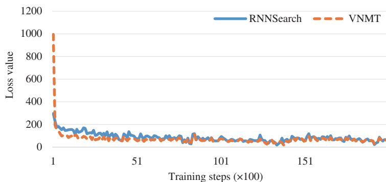
图 3 (网络版彩图) VNMT 收敛性 Figure 3 (Color online) Convergence of VNMT
