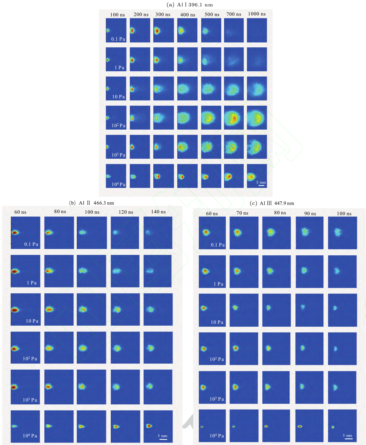
图5 0.1— 10^4 Pa 压力下, 激光能量密度为 20.8 \text{ J}\cdot\text{cm}^{-2} 时铝等离子体羽流中激发粒子的 emICCD 图像 (a) Al I (396.1 nm); (b) Al II (466.3 nm); (c) Al III (447.9 nm)
