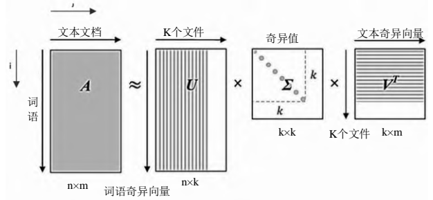
图 5 文本词语矩阵的奇异值分解
