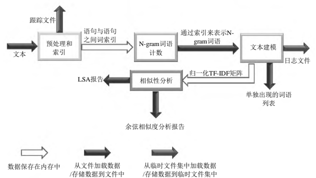
图 2 相似度估计的数据处理流程图
