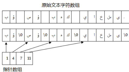
图 3 文本标记例子
