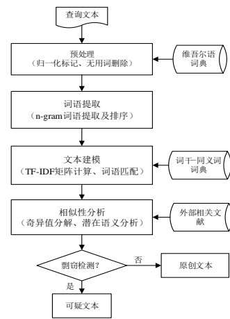
图 1 提出的文本相似度分析方法的框架
