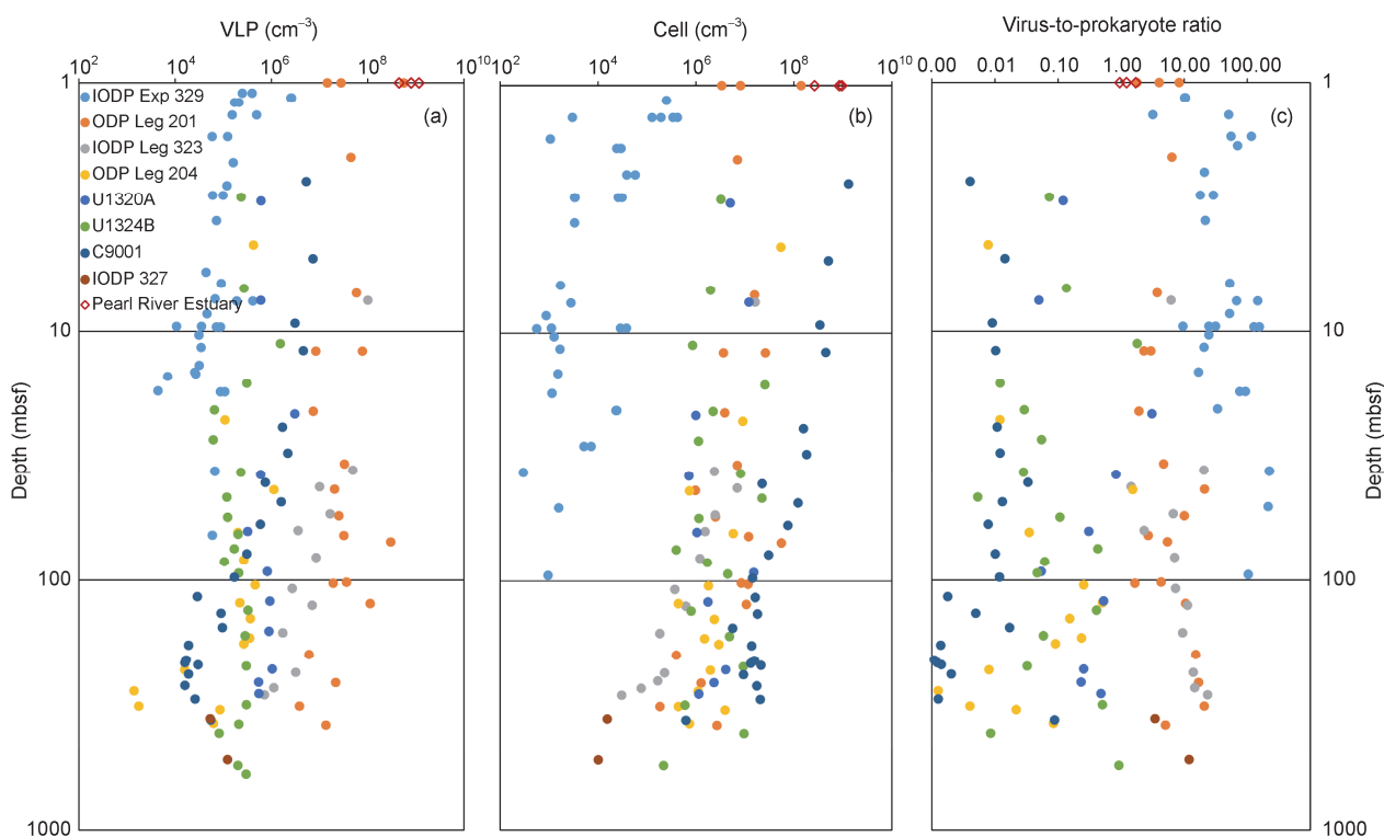
图2 深部生物圈病毒丰度(a), 原核生物丰度(b), VPR(c)的垂直分布图。数据来源: 菱形代表中国珠江口表层沉积物数据 [16] ; ODP Leg 201 [11] ; IODP Exp 329, IODP Leg 323 [13] ; ODP Leg 204, U1320A, U1324B, C9001 [12] ; IODP 327 [14]
