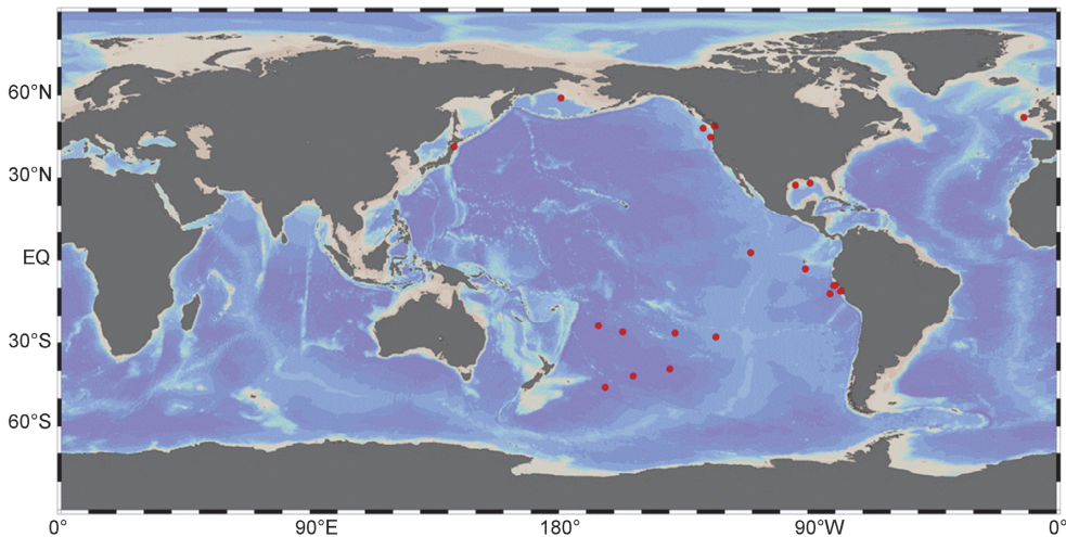
图1 深部生物圈病毒研究采样点. 航次(站位): ODP Leg 169S(1033B和1034B) [9] ; IODP 307(U1317) [10] ; ODP Leg 201(1225, 1226, 1227, 1228, 1229, 1230和1231) [11] ; IODP 329(U1365, U1366, U1367, U1368, U1369, U1370和U1371), IODP 323(U1344) [13] ; ODP Leg 204(1251), IODP 308(U1320A和U1320B) [12] ; IODP 327(1364A和1362B) [14] . 采用Ocean Data View(ODV)软件绘图
