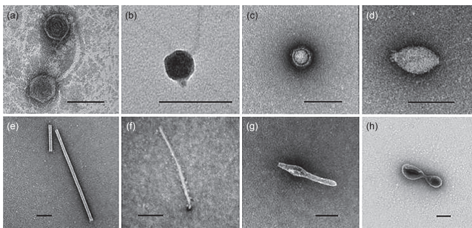
图3 玄武岩地壳热液流中的病毒形态. 钻孔U1362A样品获得的病毒电子显微镜照片(a-h), 包括相似有尾病毒目病毒(a和b), 无尾病毒(c), 类似于双尾病毒科或纺锤病毒科的柠檬状病毒(d), 类似于古病毒科的棒状病毒(e), 类似于分离自古菌的丝状病毒(f)和纺锤形病毒(g), 以及在病毒大小范围内重复观察到的二分裂结构(h), 二分裂结构不同于任何已分类的病毒形态, 可能是新型病毒或是囊泡. 标尺长度为 100 nm [14]
