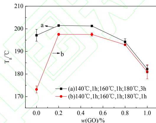
图 3 不同固化条件下动态热机械分析法得到的 GO/CF/E54-DDS 玻璃化转变温度( T_g )结果 Fig.3 The T_g results of Dynamic thermo-mechanical analysis (DMTA) of GO/CF/E54-DDS under different curing conditions
