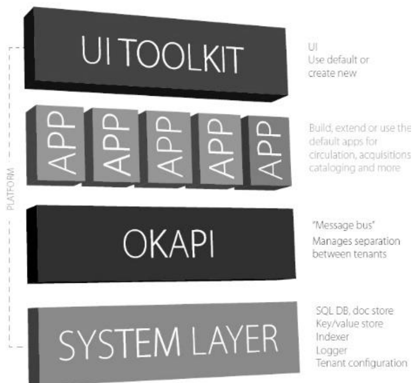
图 1 FOLIO 系统架构图
