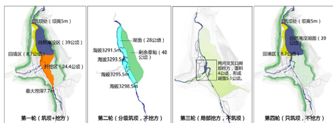
图7 鲁朗人工湖建设方案论证过程
