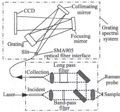
(a) 光路图
