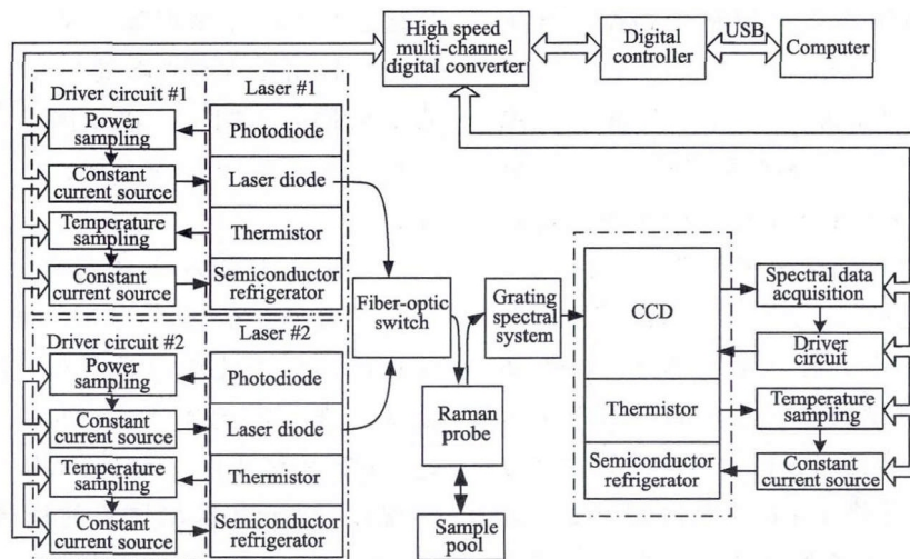
图 2 系统原理图 Fig.2 Schematic diagram of system
