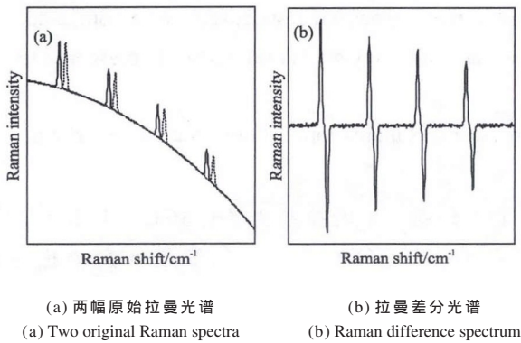
图 1 SERDS 原理图 Fig.1 Principle of SERDS
