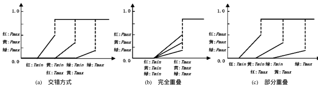
图 5 WRED 分组丢弃率
