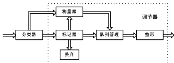
图 2 边界路由器逻辑结构
