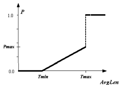
图 4 RED 分组丢弃率
