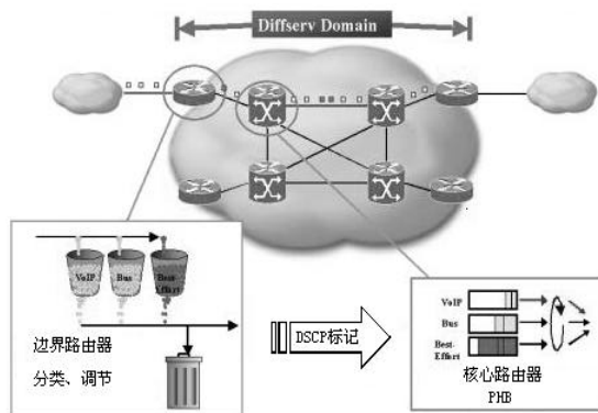
图 1 DiffServ 结构示意图
