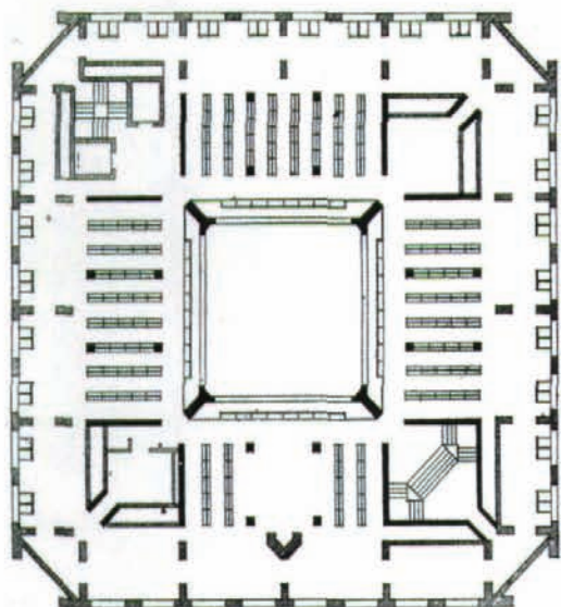
图3 菲利普斯·爱赛特尔学院图书馆平面图 (资料来源: http://www.greatbuildings.com/ )
