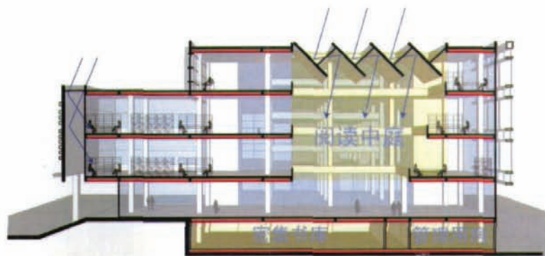
图5 南洋学院图书馆剖面之一
