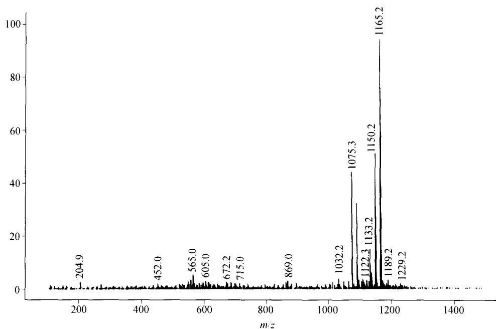
图 4 TMeQ[6]的质谱图
