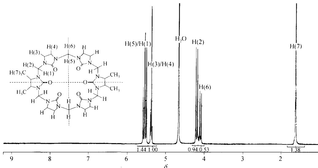
图 2 TMeQ[6]在 D 2 O 中的 1 H NMR 谱图
