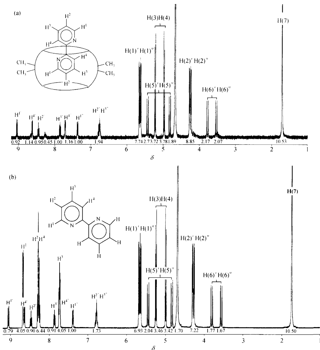
图5 TMeQ[6]与bpy · 2HCl以比例为1:1.1(a)和1:3(b)混合的 1 H NMR谱图
