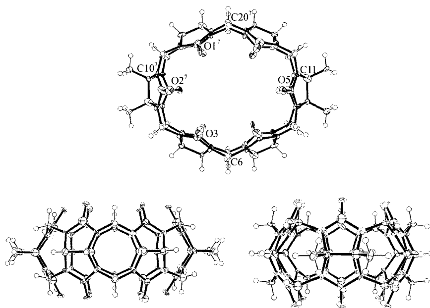
图3 TMeQ[6]的晶体结构
