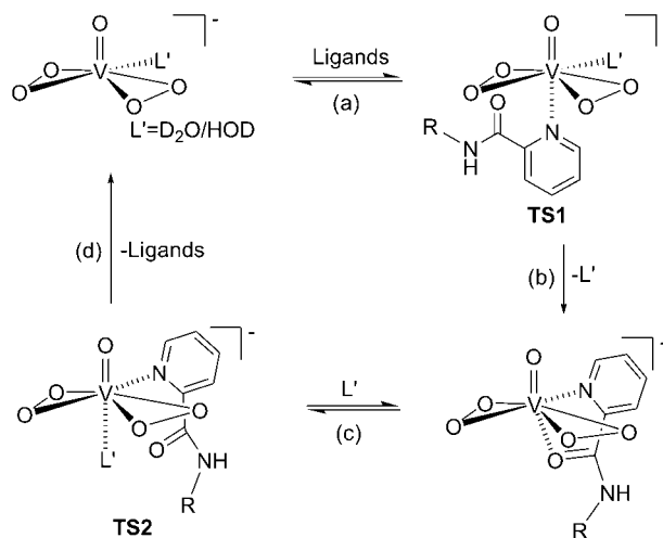
图式 2 bpV 与 N -取代皮考啉酰胺相互作用的可能模式
