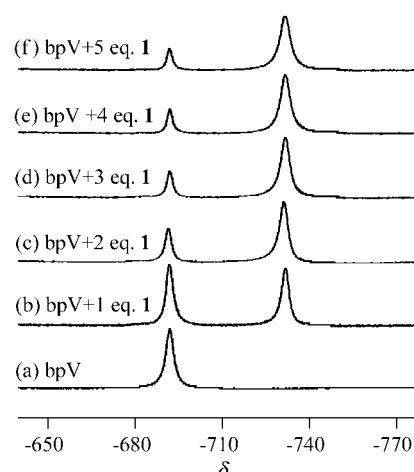
图 1 bpV 与不同摩尔比 N -甲基-皮考淋酰胺相互作用体系的 ^{51}\text{V} NMR 谱
