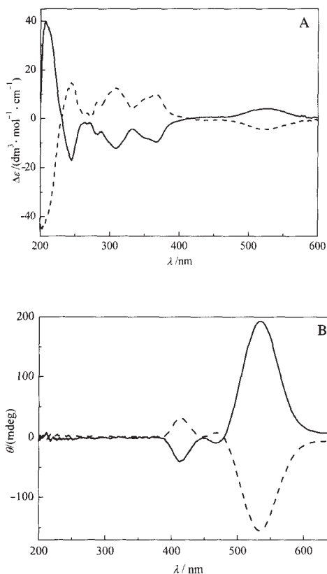
图 3 配合物 1a 和 1b 的溶液 CD(A)和固体 CD(B)光谱图 Fig.3 CD spectra of 1a and 1b in CH 3 OH solution (A) and on KCl pellets(B) 1a: dashed line, 1b: solid line
