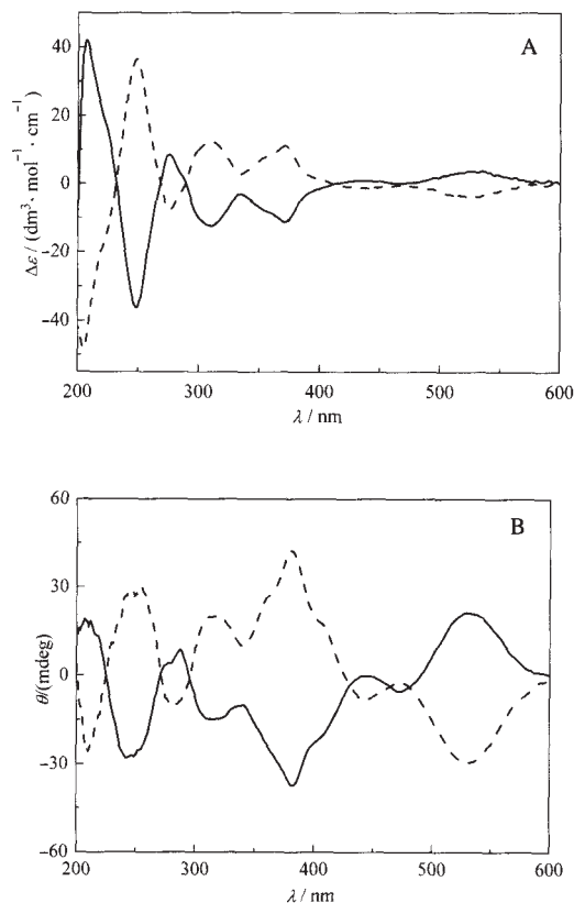
图 4 配合物 2a 和 2b 的溶液 CD(A)和固体 CD(B)光谱图 Fig.4 CD spectra of 2a and 2b in CH 3 OH solution (A) and on KCl pellets (B) 2a: dashed line, 2b: solid line
