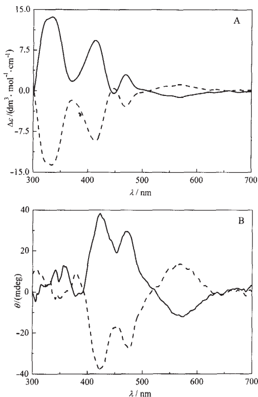
图5 配合物 3a 和 3b 的溶液 CD(A)和固体 CD(B)光谱图 Fig.5 CD spectra of 3a and 3b in \text{CHCl}_3 solution (A) and on KCl pellets(B) 3a: dashed line, 3b: solid line
