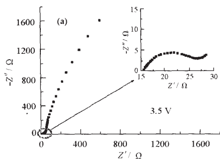
图2 尖晶石锂锰氧化物电极在首次脱锂过程中的 EIS 谱
