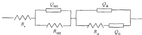
图 3 尖晶石锂锰氧化物电极在首次脱锂过程中, 电位高于 3.8 V 时 EIS 的等效电路
