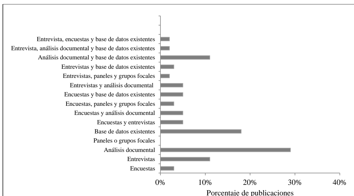
Gráfico 2. Técnicas de recolección de la información de la producción científica relacionada con contabilidad ambiental y sostenibilidad, 2013-2017.
