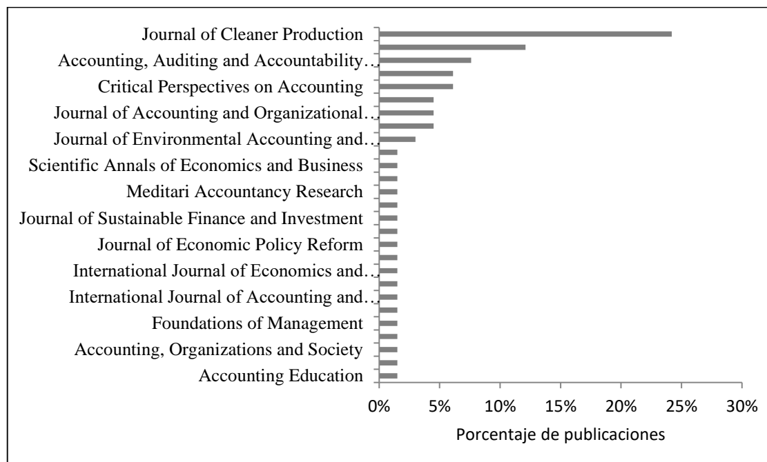
Gráfico 5. Distribución porcentual de las principales revistas con producción científica relacionada con contabilidad ambiental y sostenibilidad por número de publicaciones, 2013-2017.
