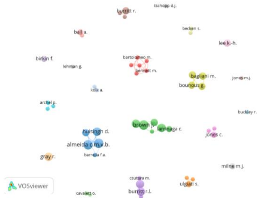
Gráfico 6. Redes de autores con producción científica relacionada con contabilidad ambiental y sostenibilidad, 2013-2017.
