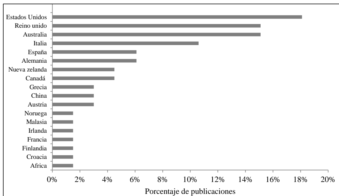
Gráfico 4. Países con producción científica relacionada con contabilidad ambiental y sostenibilidad por número de citaciones, 2013-2017.
