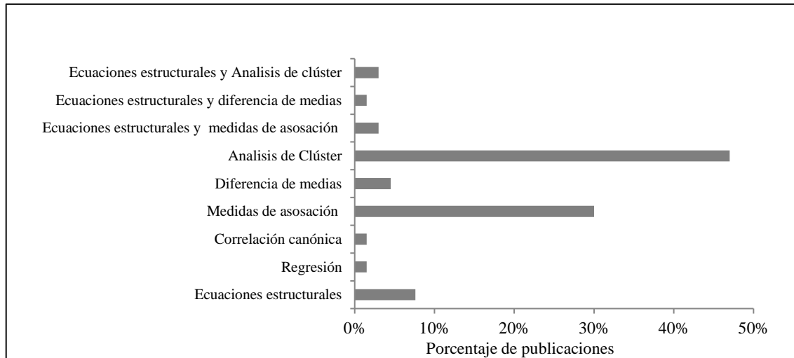
Gráfico 3. Técnicas de análisis de datos de la producción científica relacionada con contabilidad ambiental y sostenibilidad, 2013-2017.
