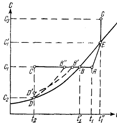
Рисунок 1.1 - Диаграмма растворимости
