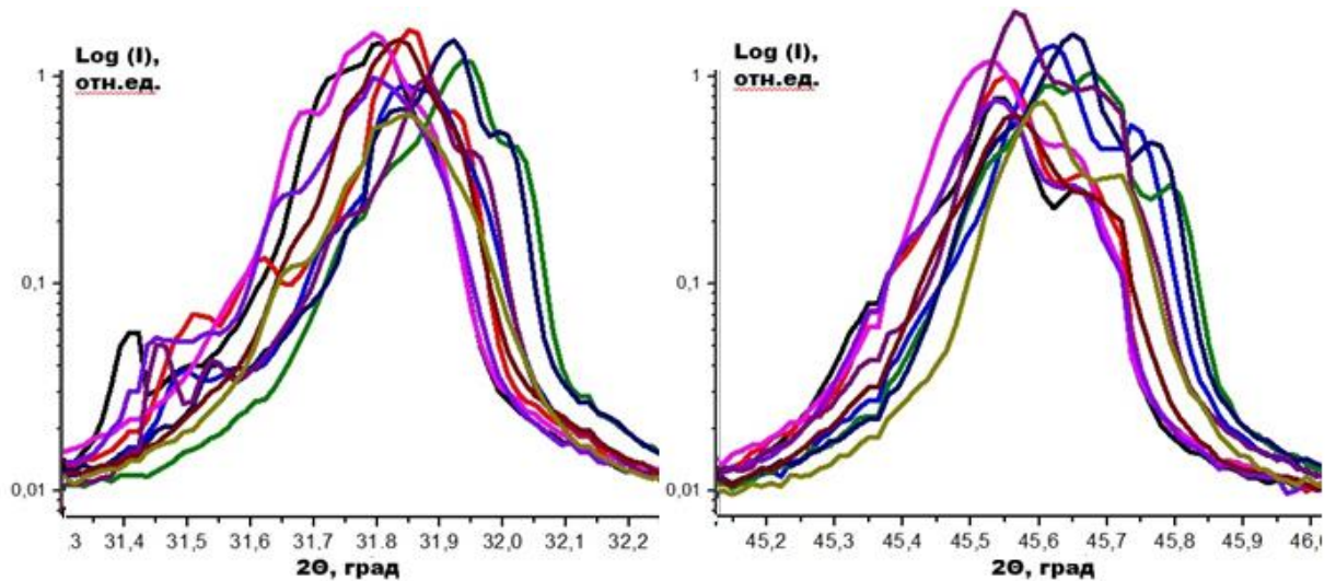
Рисунок 2.6 – первый и второй дифракционные пики с высоким разрешением по углу.
