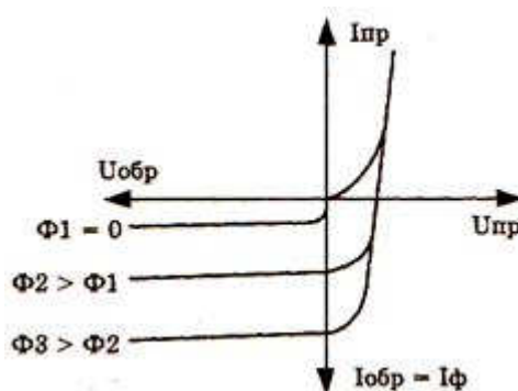
Рис. 22 ВАХ Фотодиода
