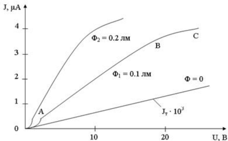
Рис. 25 ВАХ фоторезистора
