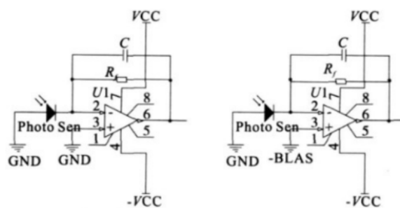
Рис. 23 Рабочая схема фотодиода
