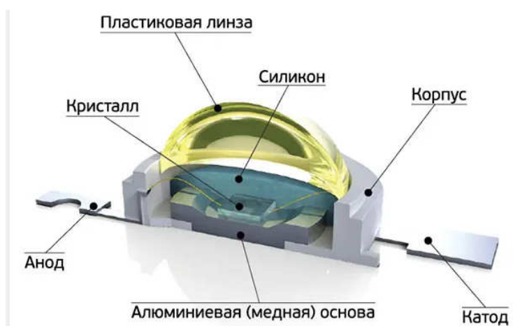
Рис.8 Устройство светодиода
