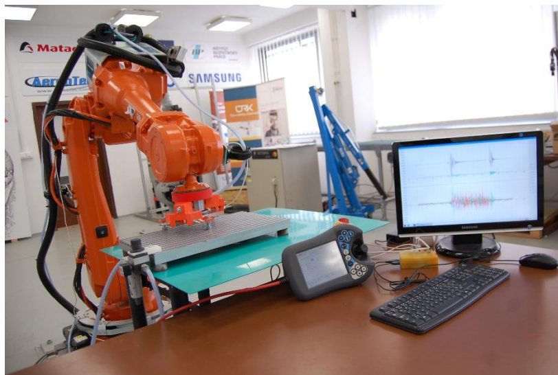
Рис. 1. Експериментальна установка
