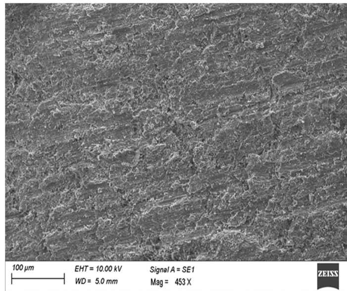
Fig. 5.a Al7075
