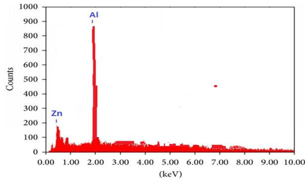
Fig. 4.a AL7075
