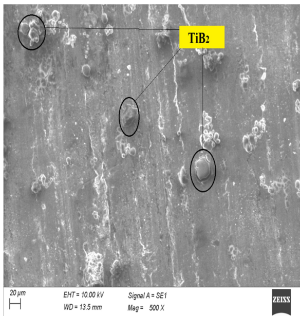
Fig. 5.b Al7075-12%TiB 2
