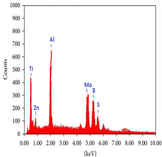
Fig. 4.d AL7075-12%TiB 2 /3%MoS 2
