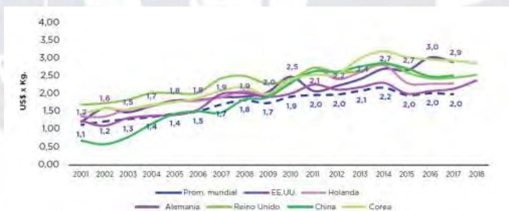
Figura 18 Precio unitario de importación anual en los principales mercados de consumo. Publicado por el Ministerio de Agricultura y Riego. Recuperado de http://agroaldia.minagri.gob.pe/biblioteca/download/pdf/tematicas/f-taxonomia_plantas/f01-cultivo/2019/Informe-uva-peruana.pdf
