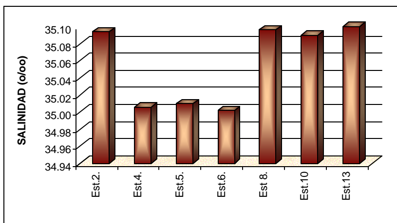
Figura Nº 11. SALINIDAD SUPERFICIAL EN EL AGUA DE MAR 14-01-00
