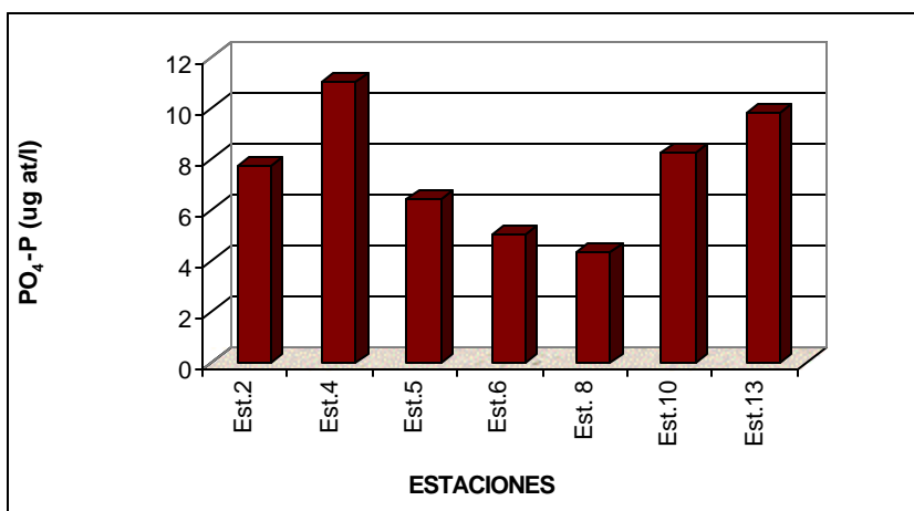
Figura Nº 30. FOSFATOS (PO 4 -P) SUPERFICIAL EN EL AGUA DE MAR 23-03-00
