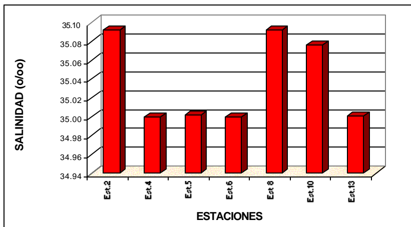
Figura Nº 14. SALINIDAD EN EL FONDO EN EL AGUA DE MAR 14-01-00
