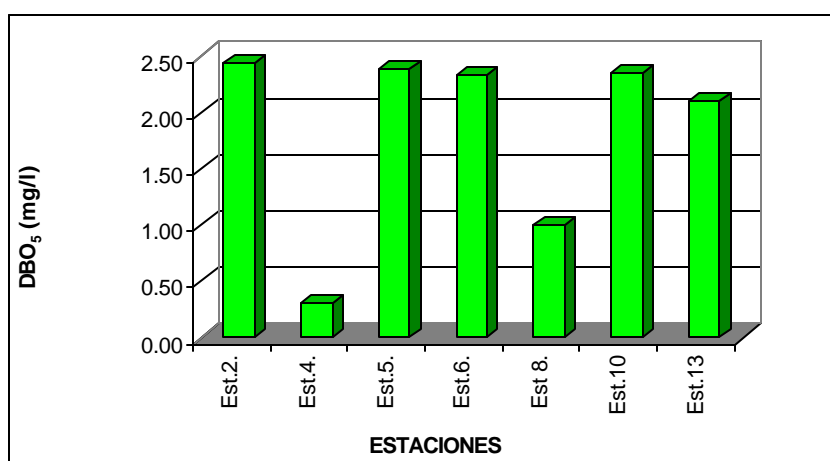
Figura Nº 23. DEMANDA BIOQUIMICA SUPERFICIAL EN AGUA DE MAR 14-01-00
