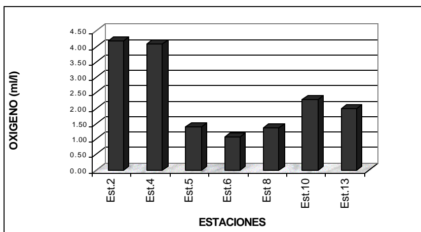
Figura Nº 20. OXIGENO DISUELTO EN EL FONDO EN EL AGUA DE MAR 14-01-00
