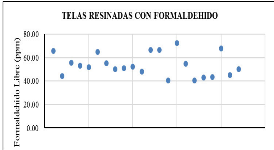
Figura 17. Formaldehido Libre en ppm como resultado del método cuantitativo.
