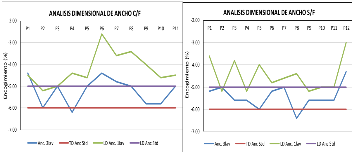
Figura 19. Comparativo de estabilidad dimensional a lo ancho de Pique 20/1 Resinado con y sin Formaldehído. Fuente: datos CK. Elaboración propia)
