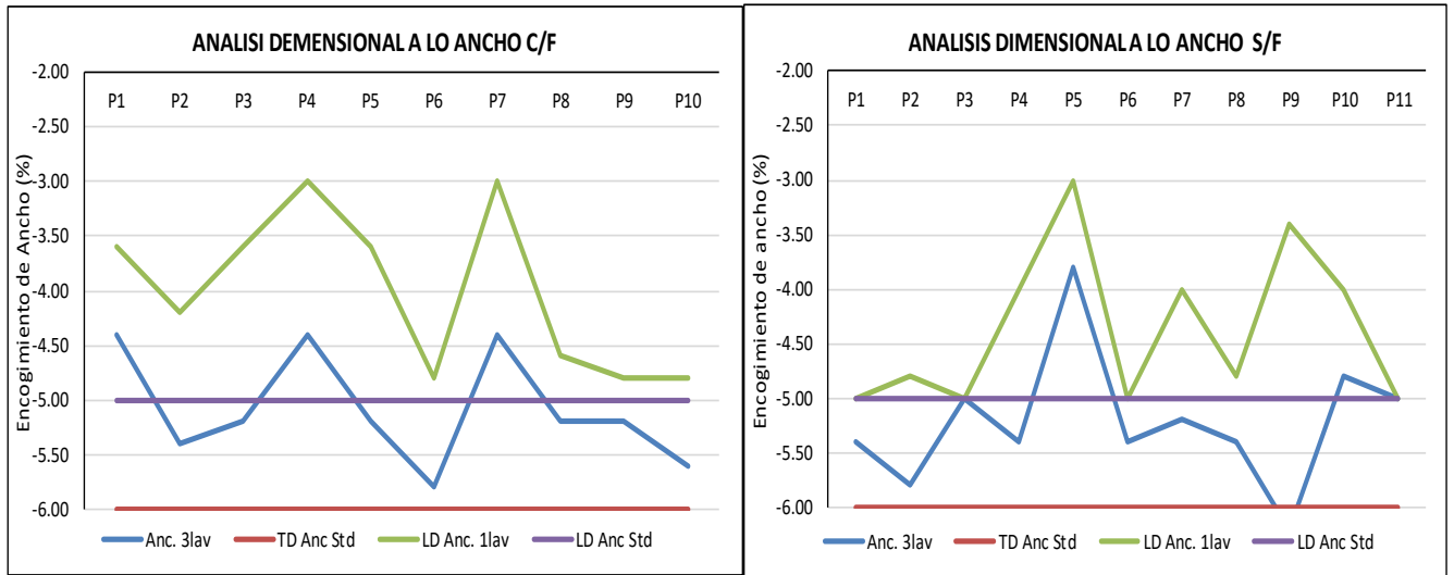
Figura 26 Comparativo de estabilidad dimensional a lo ancho de Jersey 24/1 Resinado con y sin Formaldehído Fuente: datos CK. (Elaboración propia)
