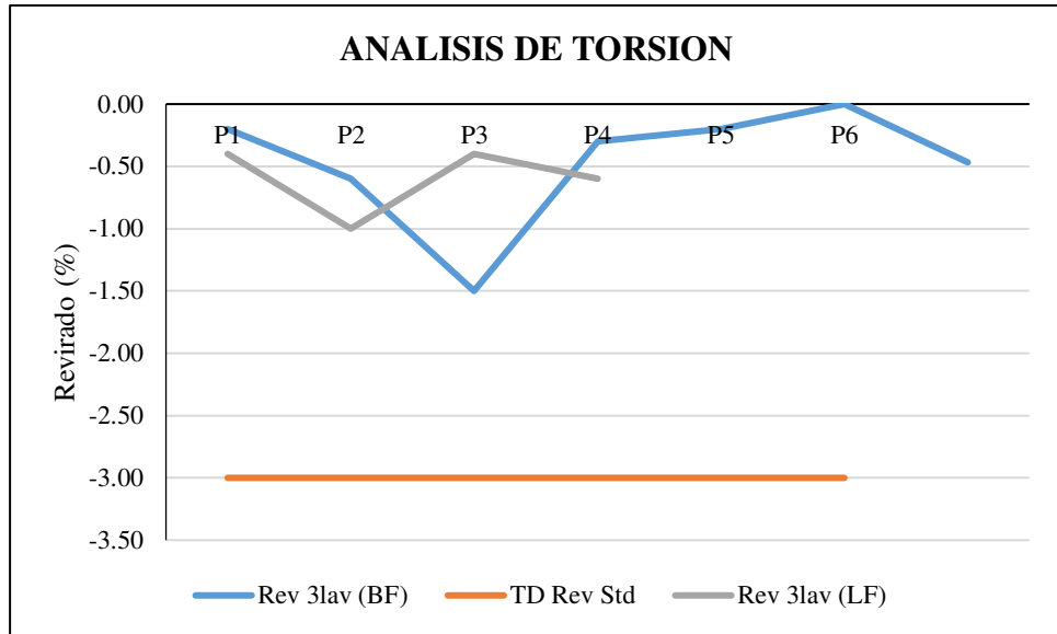
Figura 31. Comparativo de estabilidad a la torsión de Interlock 50/1 Resinado con y sin Formaldehído. Fuente: datos CK. (Elaboración propia)
