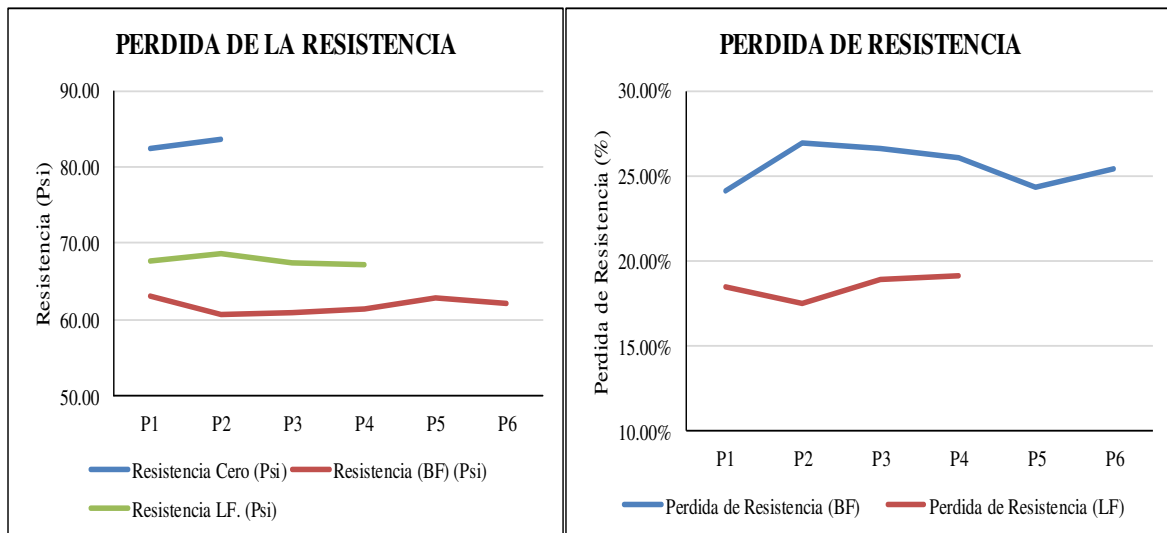
Figura 32. Análisis de pérdida de resistencia en Interlock 50/1 Resinado con y sin Formaldehído. Fuente: datos CK. (Elaboración propia)
