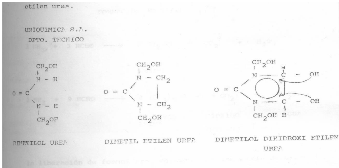
Figura 9. Dimetilol Dihidroxi Etilen Urea.
