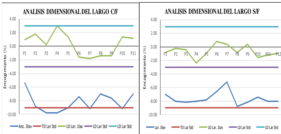
Figura 20. Comparativo de estabilidad dimensional a lo largo de Pique 20/1 Resinado con y sin Formaldehído. Fuente: datos CK. Elaboración propia.
