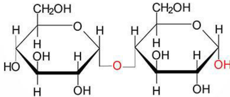
Figura 2. Anillos de Anhidro D-glucosa.
