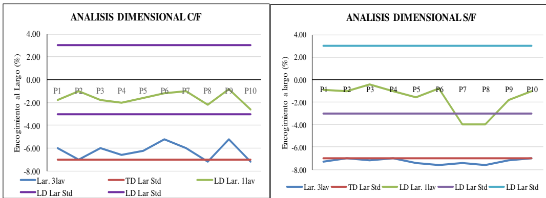
Figura 23 Comparativo de estabilidad dimensional a lo largo de Pique 50/2 Resinado con y sin Formaldehído. Fuente: datos CK. (Elaboración propia)
