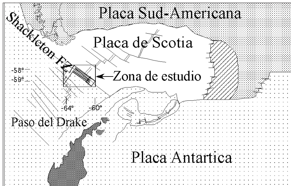
Figura 1. Situación de la zona de estudio dentro del contexto geológico del Arco de Scotia. Se muestran los principales rasgos tectónicos. Según Flores-Márquez et al. (2003a).
