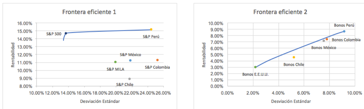
Ilustración 1: Fronteras eficientes. Fuente: Elaboración propia
