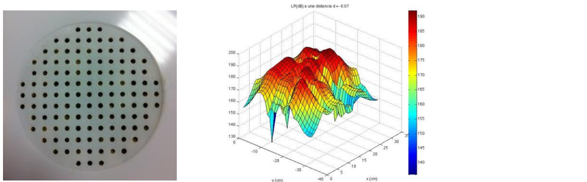
Figura 3. Holografía acústica de campo cercano (NAH) de panel perforado
