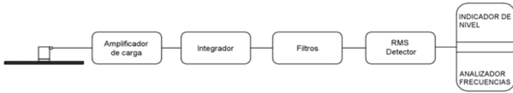
Figura 1. Esquema básico de un medidor de vibraciones con sensor de aceleración piezoeléctrico
