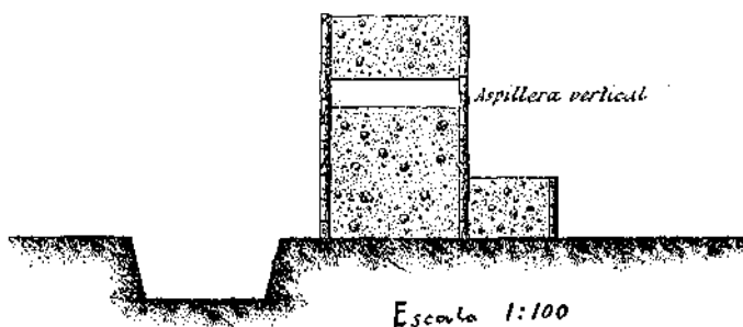
Perfil del reducto de Iba.
