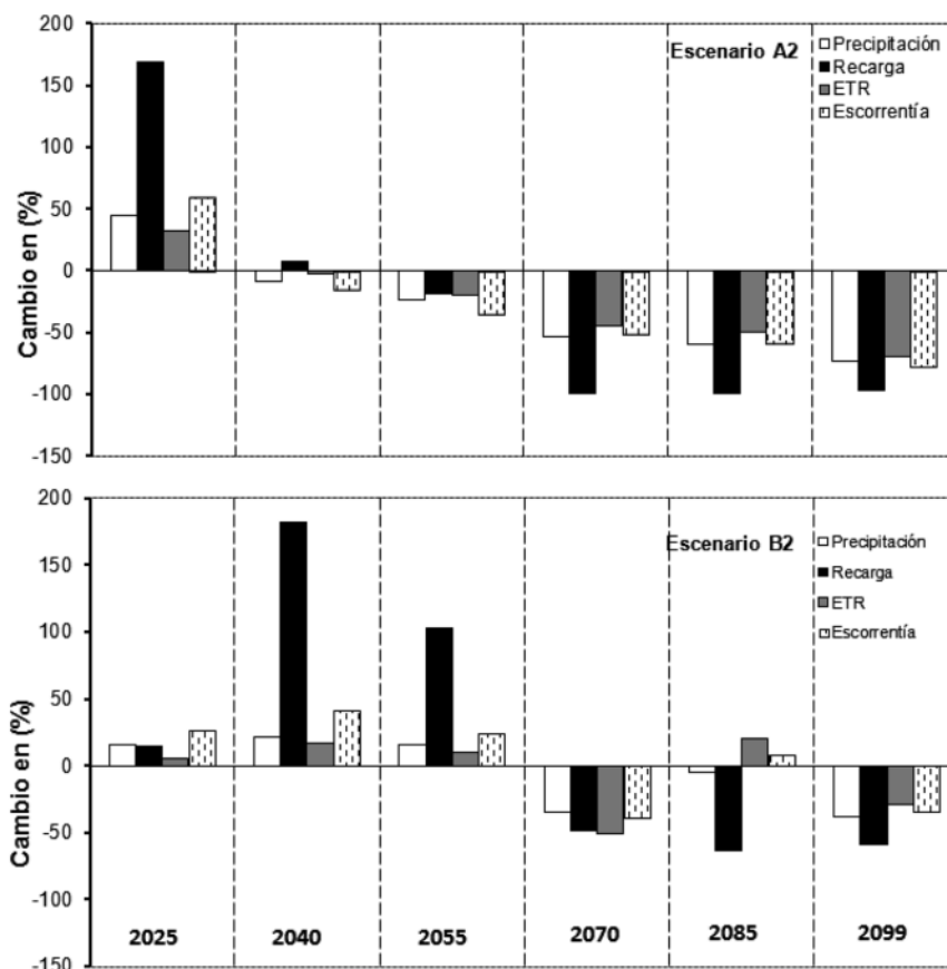
Fig. 2.- Resultados del balance de agua para los escenarios A2 (arriba) y B2 (abajo). Porcentaje anual de cambio respecto al periodo base de las variables obtenidas de Hydrobal para los años simulados. Balance del periodo base (1961-1990): P = 285,4 mm; Es = 4,39 mm; ETR = 204,7 mm, R = 32,6 mm
