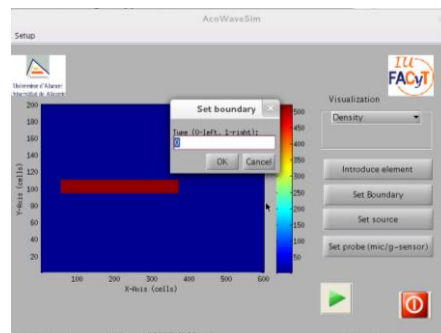
Figura 4. Pantalla principal de AcoWaveSim
