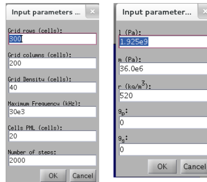
Figura 2. Menú de configuración de la malla de simulación del material a incluir.
