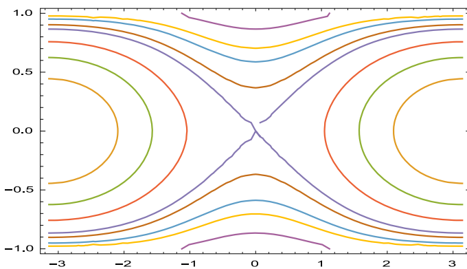
Fig. 3 Case \varepsilon > 1
