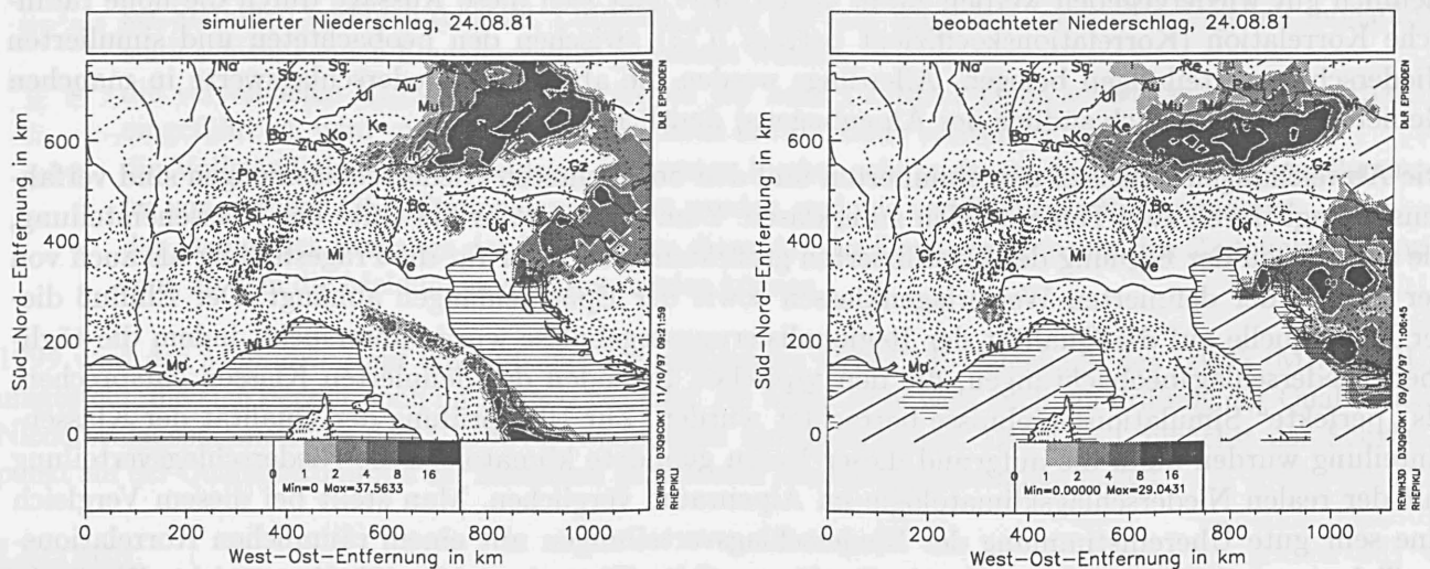
Abbildung 2: Beobachteter (rechts) und mit REWIH3D simulierter (links) Niederschlag (in mm/Tag) im Alpenraum: 24. August 1981. Im schraffierten Gebiet standen Niederschlagsmessungen nicht zur Verfügung.
