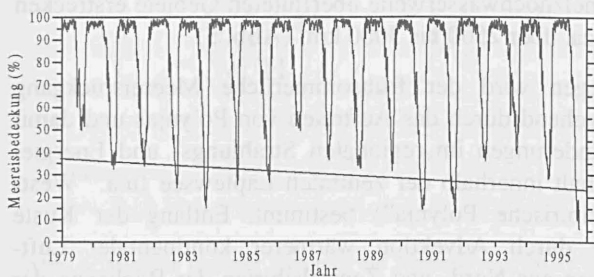
Abb. 1: Zeitlicher Verlauf (Tagesmittel) der Meereisbedeckung in der Lapteewsee von 1979 bis 1995, ferner die lineare Regressionsgerade der sommerlichen minimalen Eisbedeckung.
