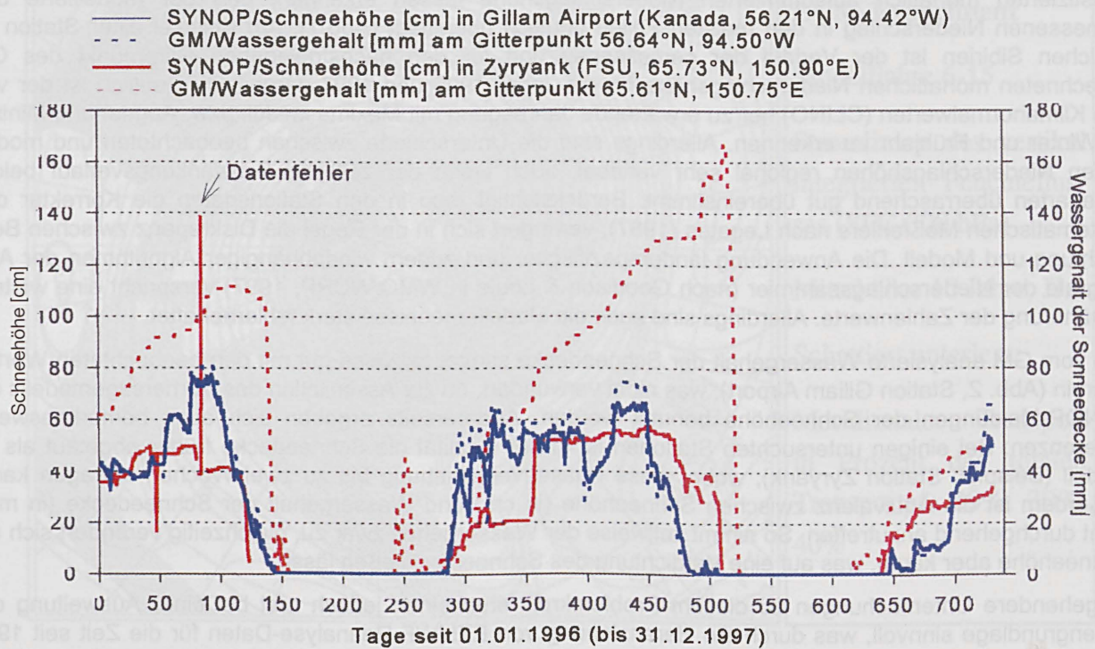
Abb.2: Vergleich zwischen beobachteter und für das Globalmodell des DWD assimilierter Schneedecken-höhe für zwei Stationen in Sibirien und Kanada, Januar 1996 - Dezember 1997.
