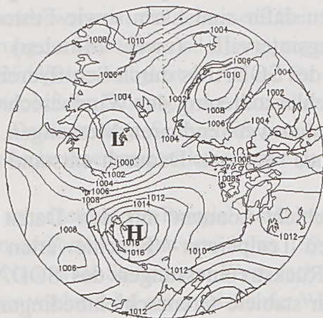
Abb. 6: Mittlerer täglicher Luftdruck auf Meeresniveau (SLP) über der Arktis für den Zeitraum 10. bis 14. Juni 1979. Abstand der Isobaren 2 hPa.
