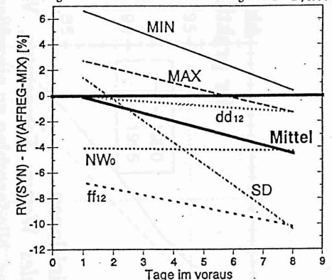
Abb. 11 Leistungsvergleich SYN und AFREG-MIX in der Mittelfristvorhersage. DWD, 1997.
