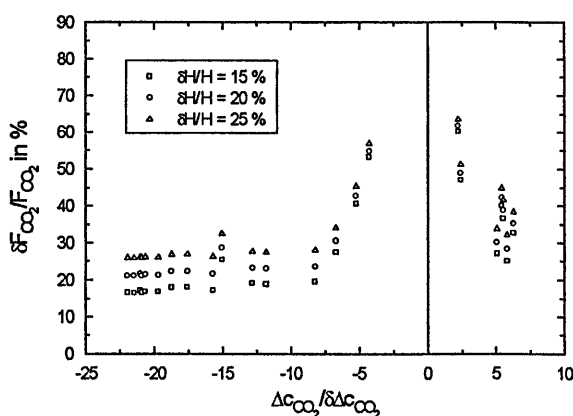
Abb. 1: Mittlerer relativer Fehler \delta F_i/F_i der RCS-Methode in Abhängigkeit von \Delta c_{\text{CO}_2}/\delta \Delta c_{\text{CO}_2} (from Kramm et al., 1998b).
