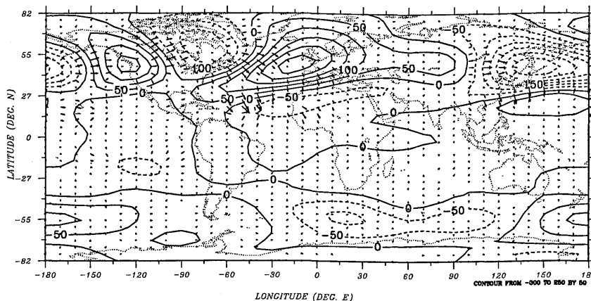
Abb.1b: Mittlere globale Verteilung des zonal asymmetrischen Geopotentials (gpm) sowie der horizontalen Komponenten des entsprechenden Plumb-Vektors, wobei die maximale Pfeillänge 47,2 \text{ m}^2/\text{s}^2 beträgt, für Januar von 1979-92 der 300 hPa Fläche.
