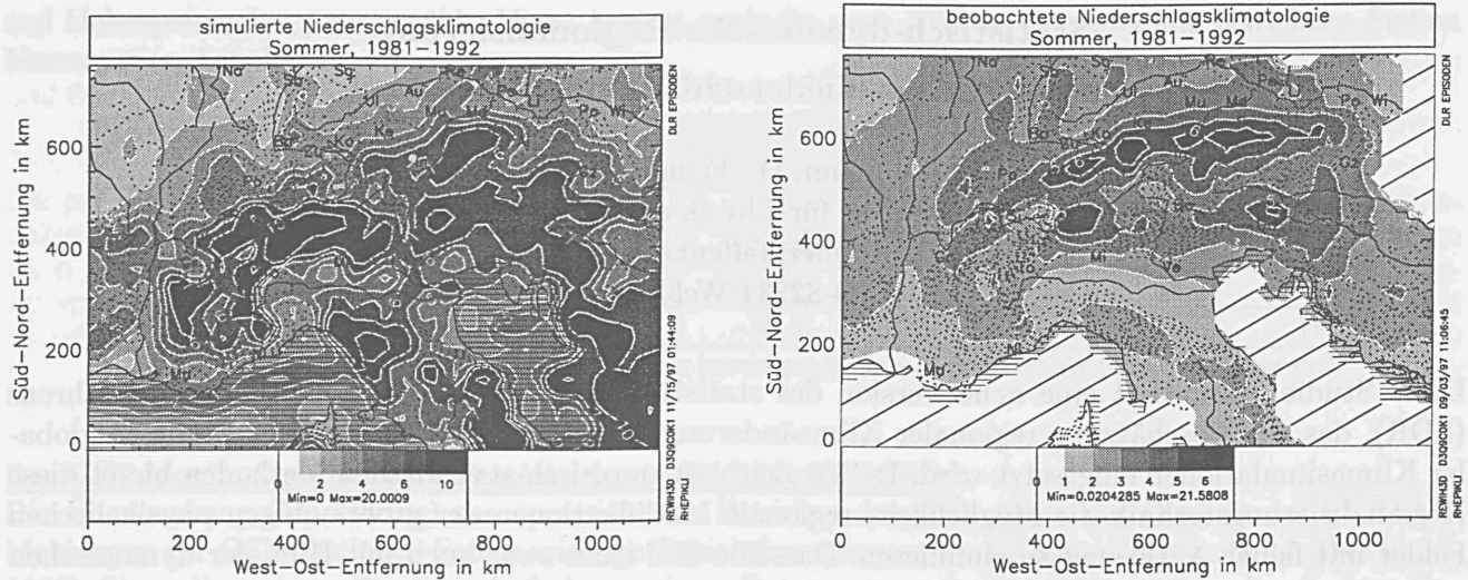
Abbildung 1: Sommerliche Niederschlagsklimatologie (Jahre 1981-1992, in mm/Tag) im Alpenraum. Links: simulierte, rechts: beobachtet. Im schraffierten Gebiet standen Niederschlagsmessungen nicht zur Verfügung.
