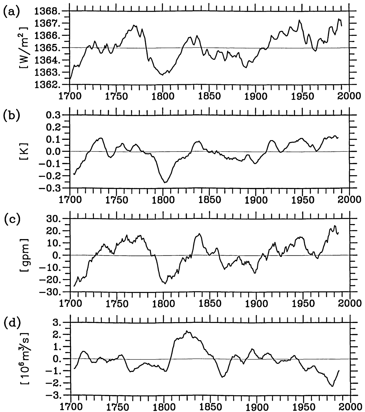
Abbildung 1: Aus der vorgeschriebenen solaren Einstrahlung nach Hoyt und Schatten (1993) (a) resultierende Anomalien der global gemittelten bodennahen Lufttemperatur (b), der zwischen 20^{\circ}\text{N} und 37^{\circ}\text{N} gemittelten geopotentiellen Höhe in 30 hPa (c) und des Maximums der meridionalen Stromfunktion im Atlantik (d). Die Zeitreihen in (b), (c) und (d) stellen die mittleren Differenzen der beiden Realisationen zum entsprechenden Kontrolllauf mit konstanter solarer Einstrahlung von 1365 \text{ W/m}^2 dar. Die Zeitreihen wurden über 9 Jahre gleitend gemittelt.
