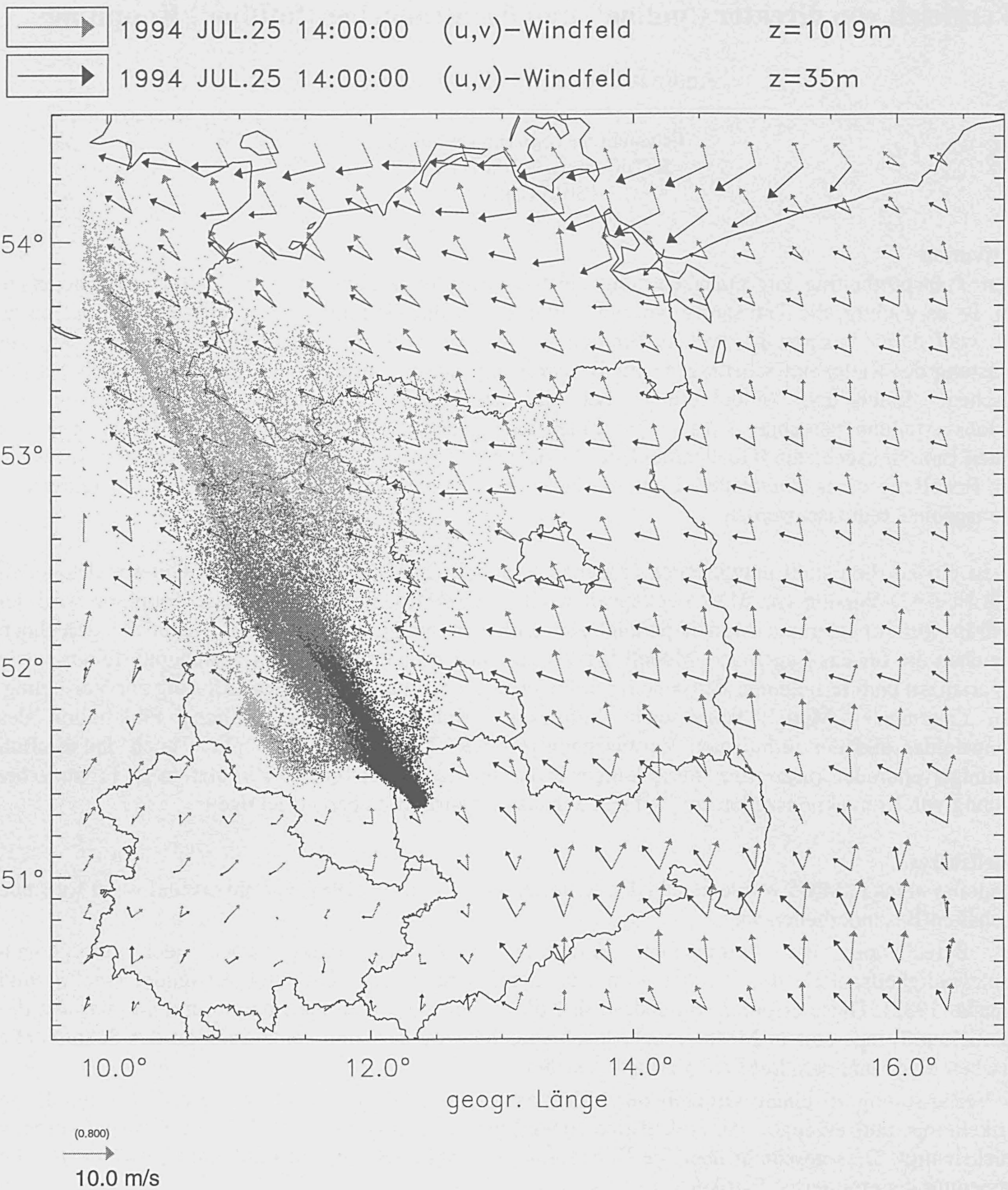
Abb.1: Partikelpositionen nach 16 Stunden Emission aus dem Raum Leipzig (Startzeit: 25. Juli 1994, 10 UTC) aufgeteilt in drei Altersklassen (Graustufe der Partikel wechselt alle 320 Min.). Ferner sind an jedem vierten Gitterpunkt von MM5 ( \Delta x = \Delta y = 6 km) die Vektoren des Horizontalwindes für 14 UTC in der ersten (schwarz) und der sechsten Schicht (grau, Schichtmitten in 35 und 1019 m) angezeigt. Zur Orientierung wurden zusätzlich die Grenzen der neuen Bundesländer und die Küste eingezeichnet.
