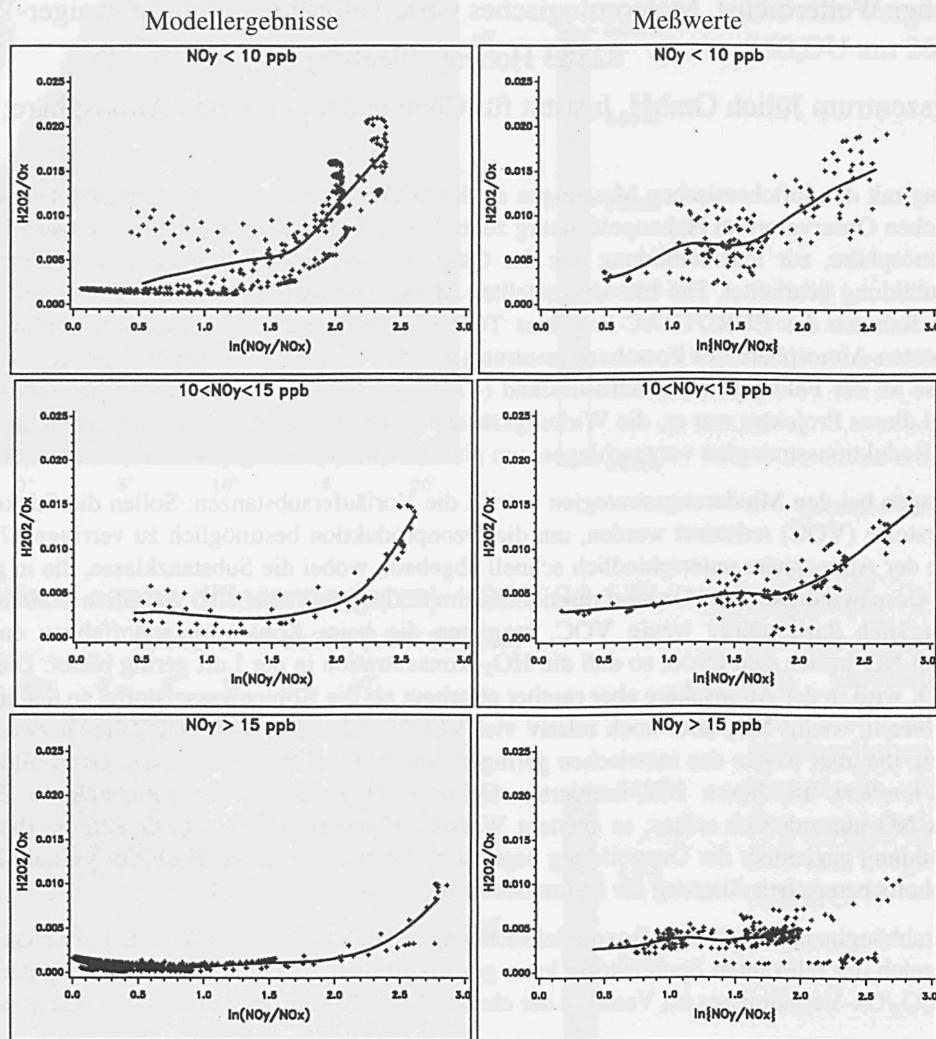
\text{H}_2\text{O}_2/\text{O}_x -Verhältnis in Abhängigkeit des chemischen Alters, sortiert nach verschiedenen \text{NO}_y -Klassen.
