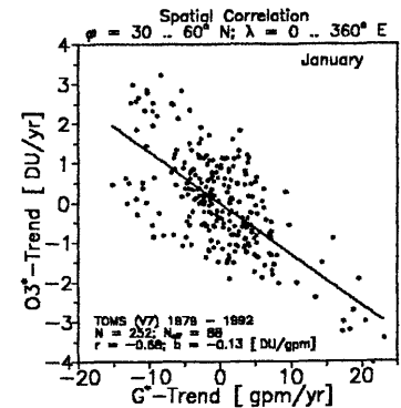
Abb. 2: Korrelogramm der Gitterpunktwerte der Abb. 1 a und b. * = Abweichung vom zonalen Mittelwert.
