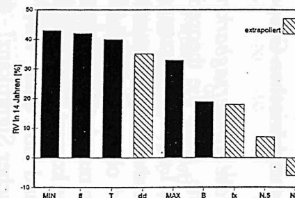
Abb. 8 Fortschritte (RV in 14 Jahren) in der kurzfristigen Wettervorhersage (DWD, Prognostiker, 4/84 - 12/97). B = Bedeckungsgrad; N.0, N.5 = Niederschlag/12 Stunden mit Schwelle 0 bzw. 0.5mm (hier TSS-Differenzen!)
