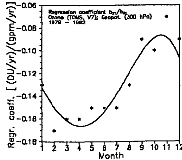
Abb. 4: Jahresgang des Regressionskoeffizienten zwischen zonal asymmetrischen Geopotential- und Ozontrend
