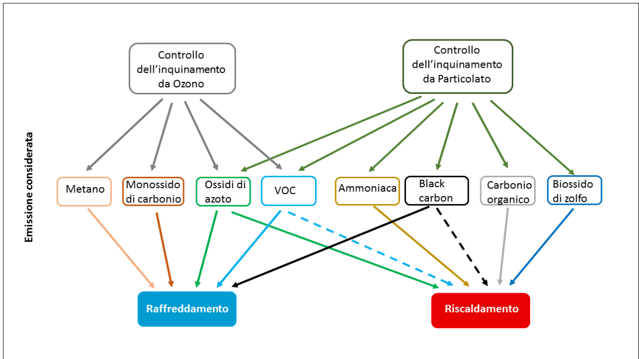
Figura 1: Diagramma schematico dell'azione di controllo su specifiche emissioni e impatto sul clima. Le linee solide rappresentano l'impatto noto, quelle tratteggiate indicano impatto incerto. Rielaborata da [6].
