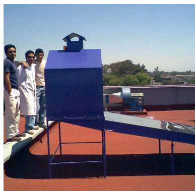
Figura 11.- Secador Solar
