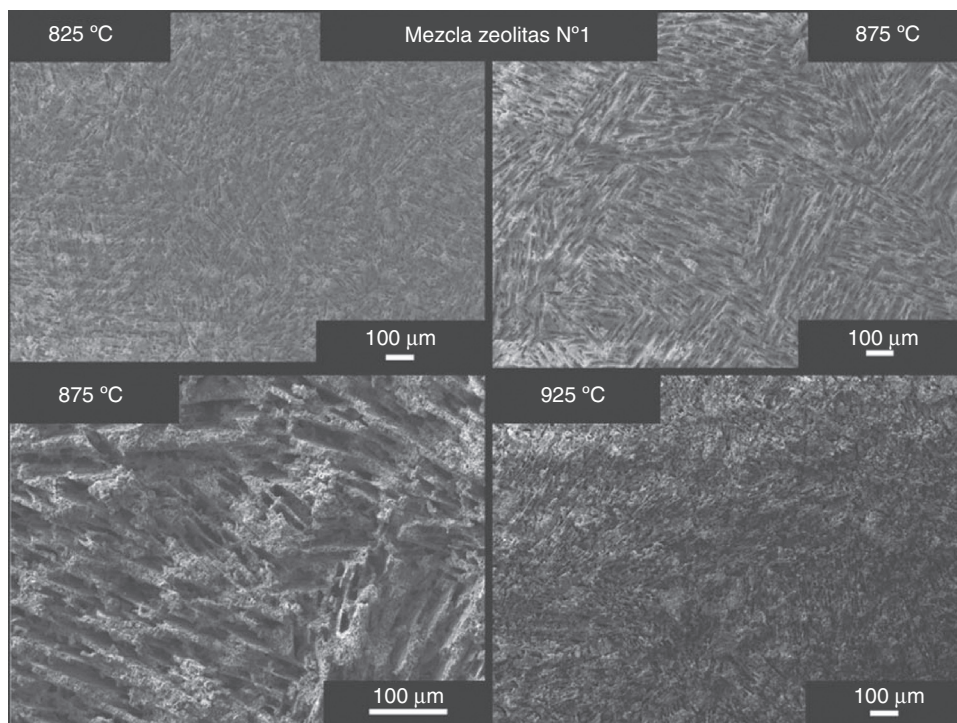
Figura 4 – Imágenes SEM de la microestructura interna de las piezas de mezcla de zeolitas número 1 (60% HA/ \beta -TCP, 20% BG 1393 y 20% ZSM-5) sinterizadas a diferentes temperaturas.
