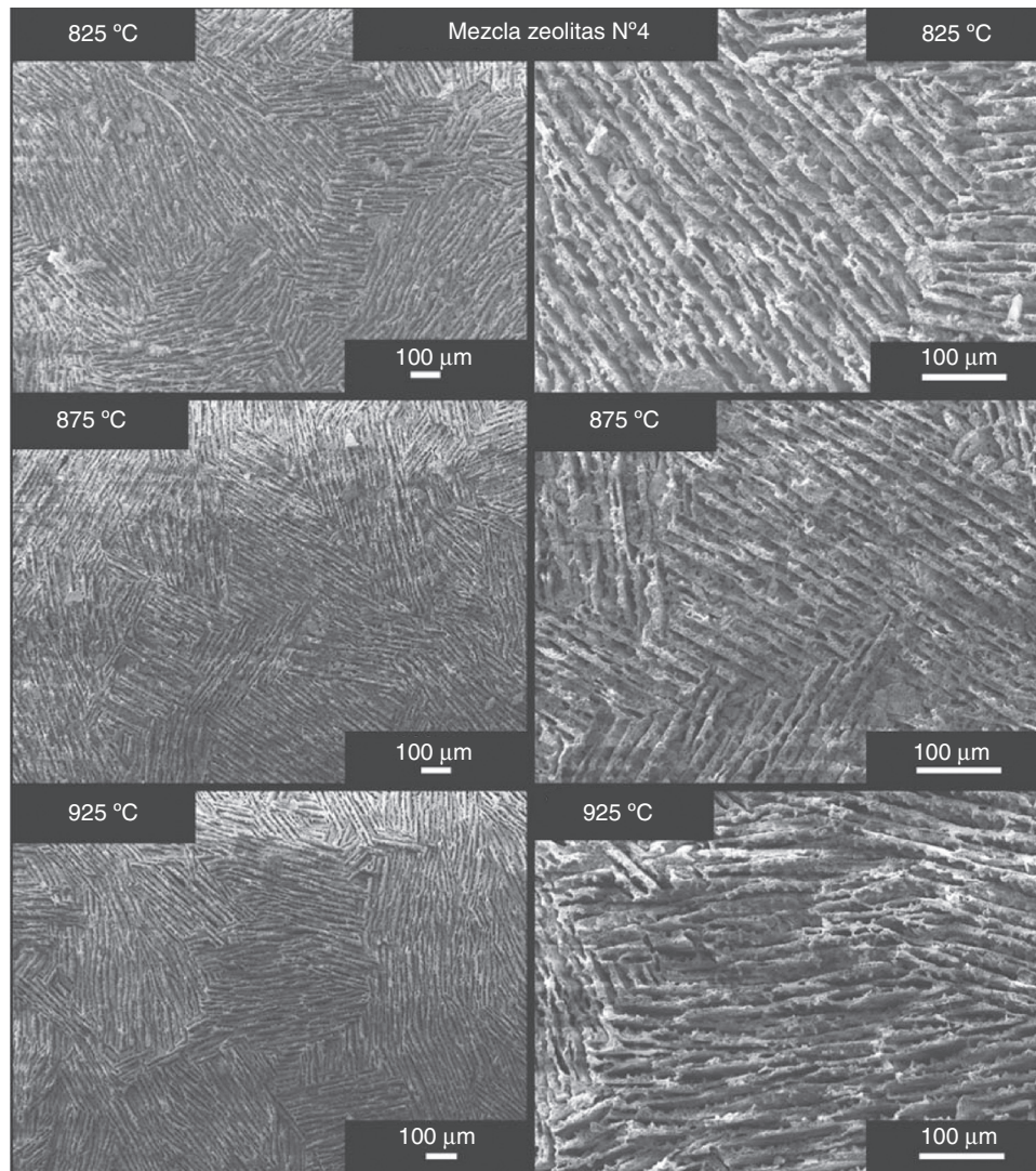
Figura 7 – Imágenes SEM de la microestructura interna de las piezas de mezcla de zeolitas número 4 (50% HA/ \beta -TCP, 30% BG 1393 y 20% en peso ZSM-5) sinterizadas a diferentes temperaturas.
