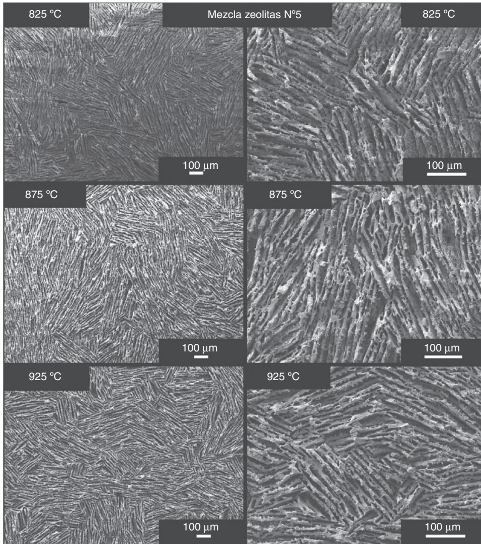
Figura 8 - Imágenes SEM de la microestructura interna de las piezas de mezcla de zeolitas número 5 (40% HA/ \beta -TCP, 30% BG 1393 y 30% en peso ZSM-5) sinterizadas a diferentes temperaturas.
