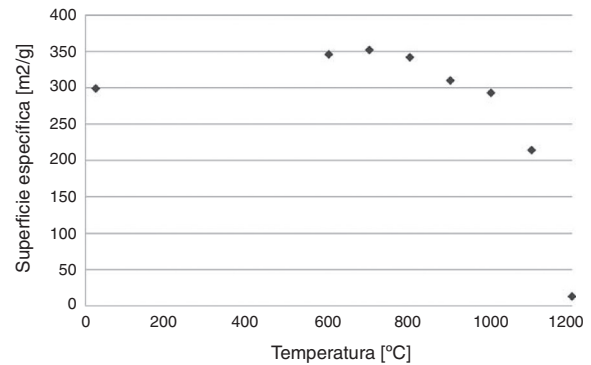
Figura 2 – Variación de la superficie específica de las zeolitas ZSM-5 después de ser sometidas a las correspondientes temperaturas hasta 1.200 °C. El primer punto corresponde con el material sin ser tratado térmicamente.
