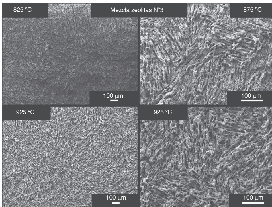
Figura 6 – Imágenes SEM de la microestructura interna de las piezas de mezcla de zeolitas número 3 (50% HA/ \beta -TCP, 25% BG 1393 y 25% en peso ZSM-5) sinterizadas a diferentes temperaturas.
