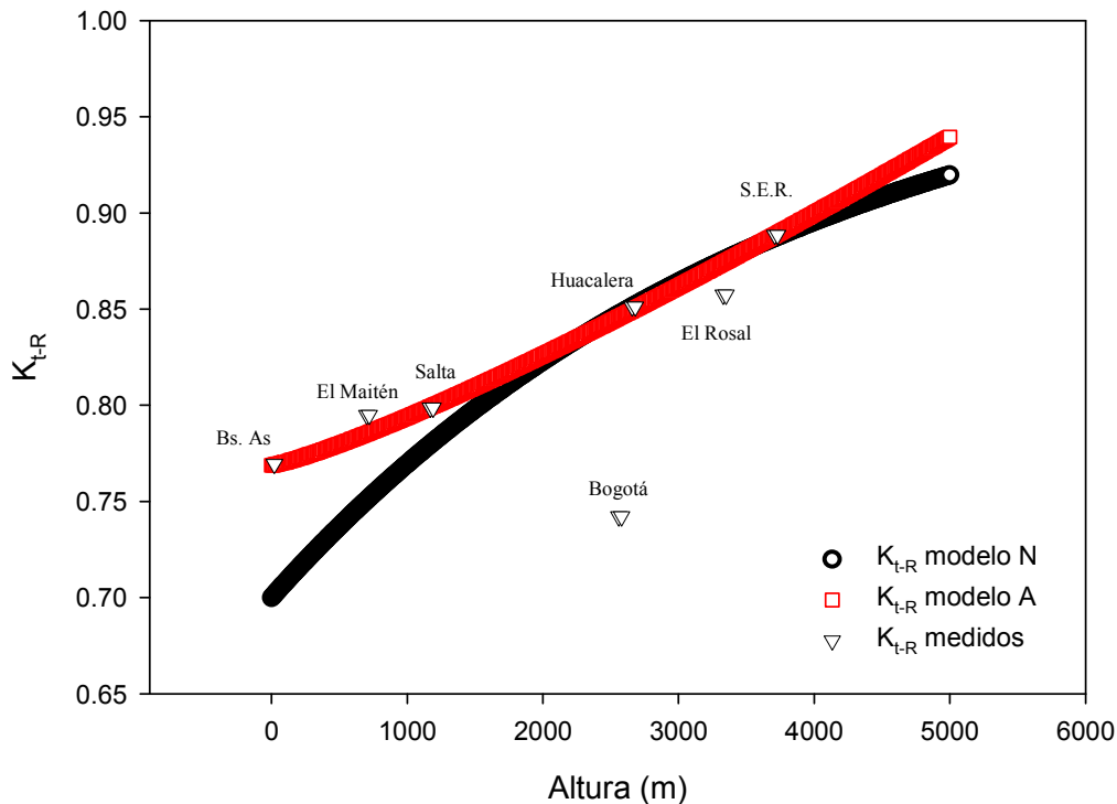
Figura 2. Posición de los índices representativos calculados para cada sitio estudiado, respecto de los modelos A y N.
