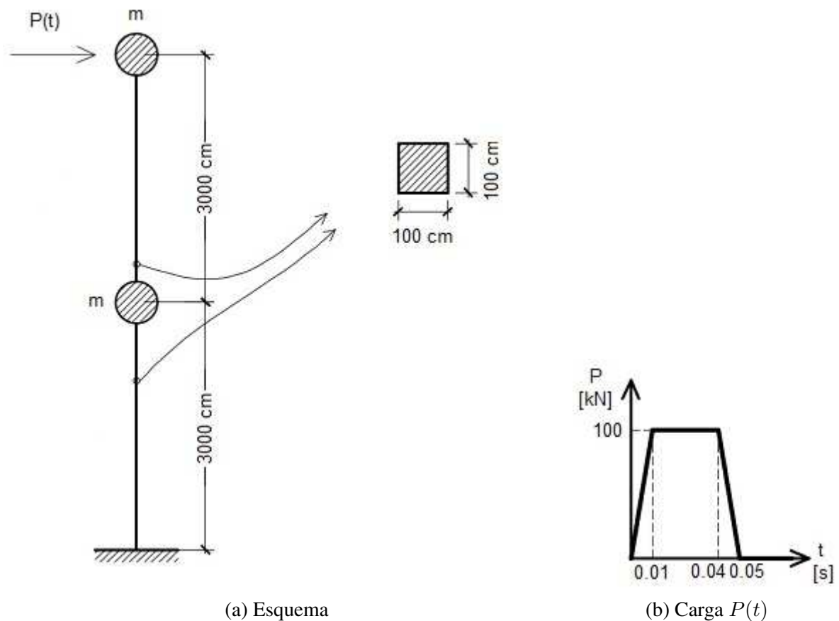
Figura 8: Modelo del primer ejemplo de análisis
