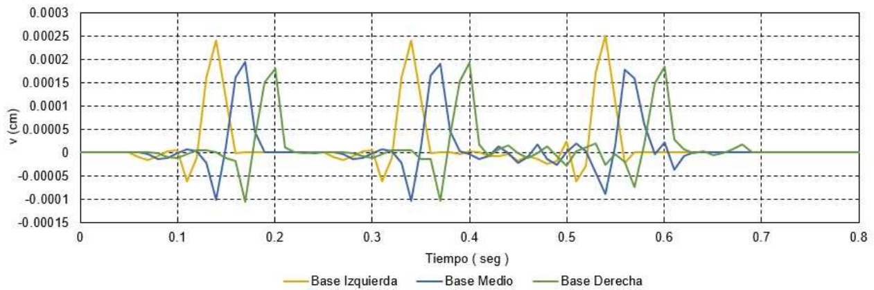
Figura 25: Desplazamiento impuesto vertical en bases
