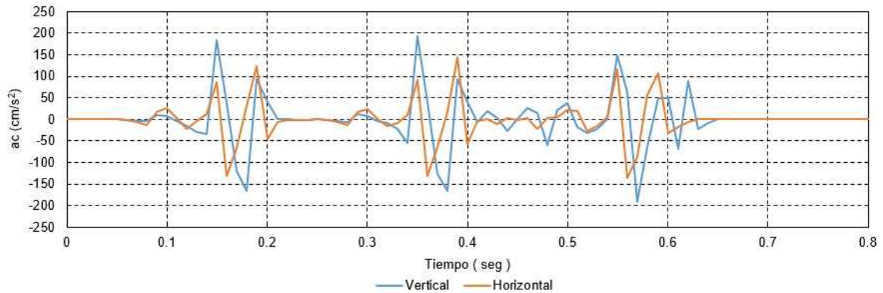
Figura 26: Acelerogramas
