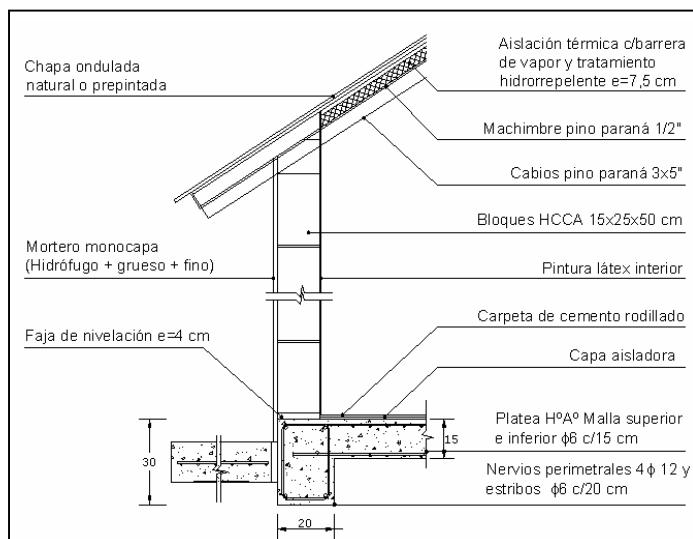
Figura 2: Corte constructivo de la vivienda
