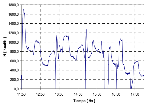
Figura 9.- Potencia desarrollada por el sistema de climatización
