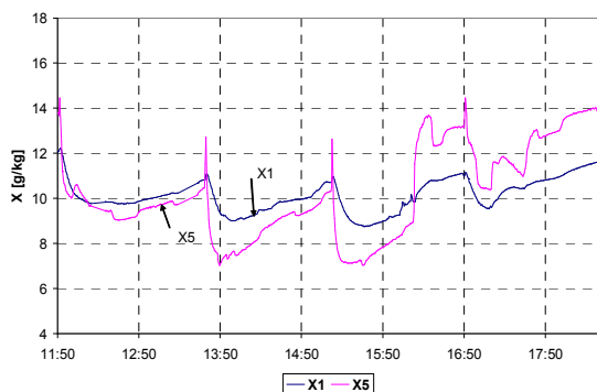
Figura 8.- Humedades absolutas dentro del local y a la salida del sistema de climatización
