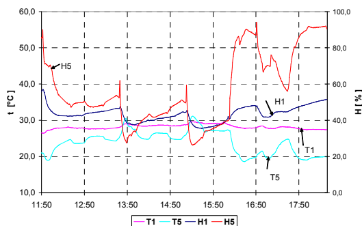
Figura 7.- Temperaturas y humedades relativas dentro de la habitación y a la salida del sistema de climatización
