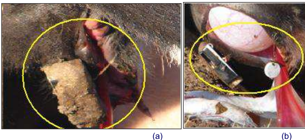
Figura 8. Sensor instalado antes del inicio de parto (a). Sensor activado al inicio del parto (b).
