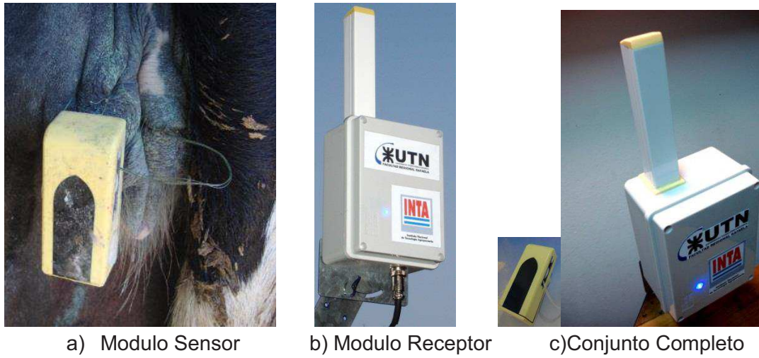
Figura 21. Distintos componentes del prototipo.
