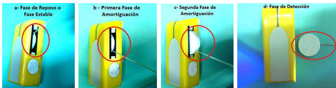
Figura 15. Fotografías del Dispositivo con detalle de Fases de Operación
