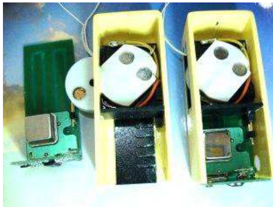
Figura 10. Vista del dispositivo sensor sin la tapa inferior transmisor y circuito electrónico decodificador
