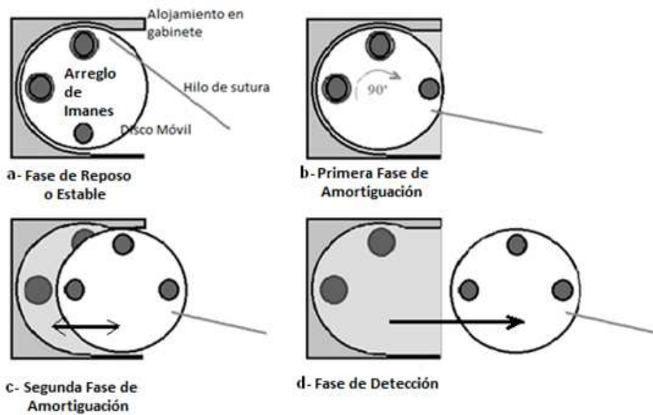
Figura 13. Esquema del dispositivo en Corte Longitudinal con detalle de Fases de Operación
