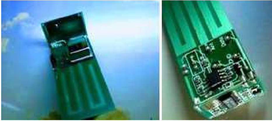
Figura 11. Detalle de antena impresa con módulo
