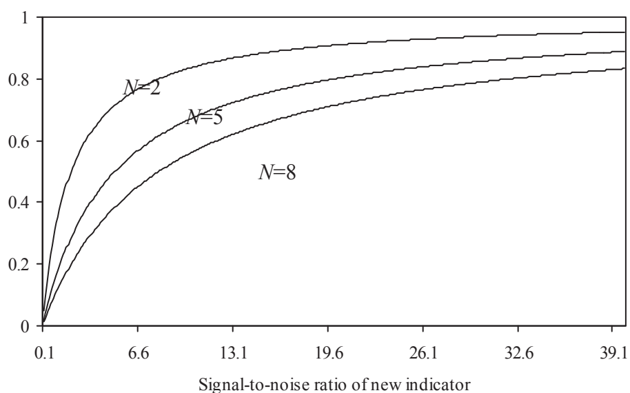
Figure 1. KL divergence
