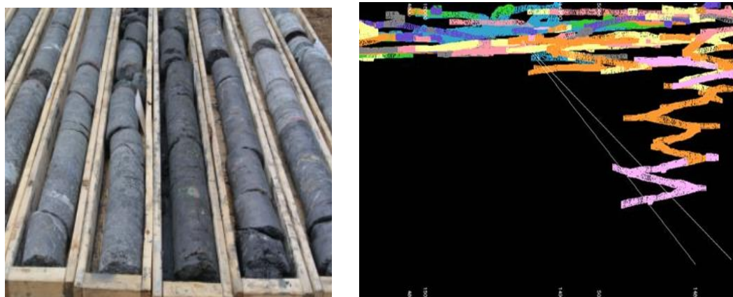
Figura 11- Filito nos testemunhos de sondagem Nível 326 GPN Fonte: Votorantim Metais
