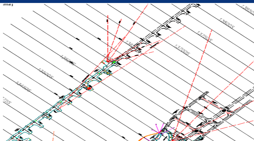
Figura 12 – Perfil Geológico Nível 326 GPN Fonte: Votorantim Metais
