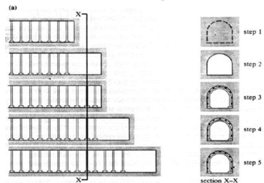
Figura 5 – Sistema de cambotas metálicas Fonte: Dimensionamento e suporte de aberturas subterrâneas
