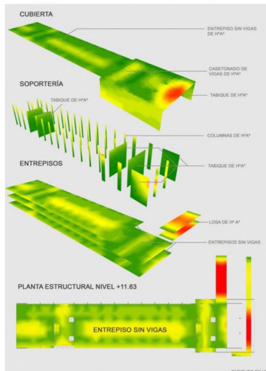
Figura 11. Concurso “Complejo Tribunal en Necochea” Diseño Estructural Paramétrico: Ing. J.Farez - Arq. P.Lordella
