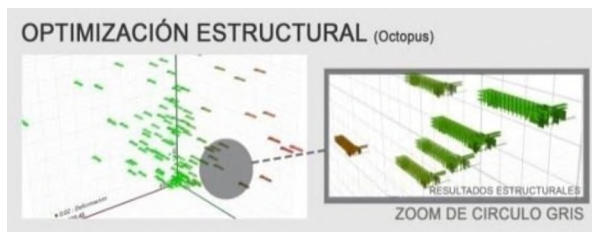
Figura 10. Proceso de optimización
