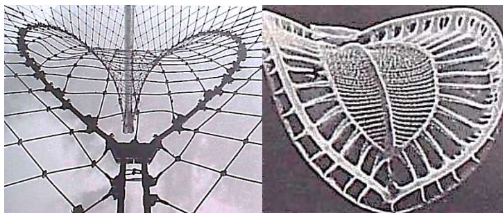
Fig. 18 – Tenso estructura de Frei Otto comparada con una diatomea vista al microscópio.
