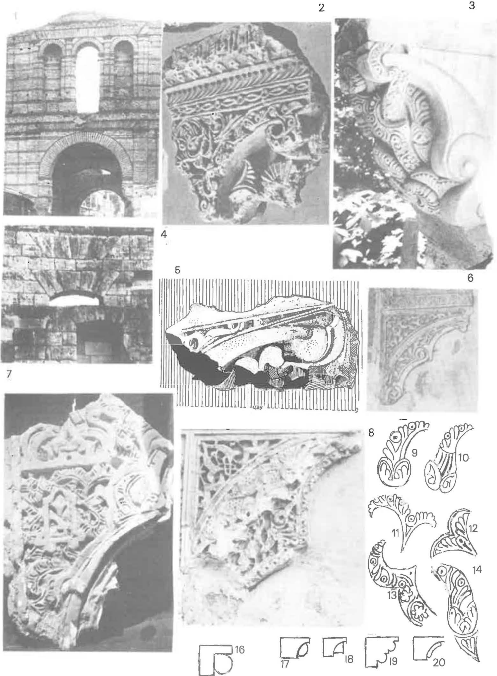
Fig. 9. 1, dinteles con dovelas de ladrillo, Anfiteatro de Burdeos; 2, ménsula de yeso, "El Castillejo", Murcia (s. XII); 3, ménsula de Biharramba = Orejas; 4, dinteles con dovelas de piedra, Anfiteatro Le Jem, Túnez; 5, piedra de ménsula encontrada en la Alhambra; 6, ménsula del Generalife; 7, ménsula encontrada en la Alcazaba de Sevilla (ss. XII-XIII); 8, ménsula del Generalife, Palmetar ; 9, pila de Marraquech (ss. XI-XII); 10, Mezquita de la Kutubiyya , Marraquech (s. XII); 11, pila marroquí (ss. XI-XII); 12-13-14, puerta Biharramba = Orejas, in costas de arcos ; 16, gorroneas de Córdoba omeya, Alcázar de Almería y Castillo de Alcalá la Real, Jaén; 17, puerta Alcazaba de los Udaya , Rabat, alminar de la Mezquita de San Sebastián, Ronda, puertas del Vino, de la Justicia y de Siete Suelos de la Alhambra, y puertas atarazanas de Málaga; 18, Alcazaba de los Udaya , Rabat, Chella y puerta de Magabar de Ronda; 19, puerta de Sevilla, Carmona; 20, puerta del Sol, Toledo, puertas de Niebla y Castillo de Véjer de la Frontera, Cádiz
