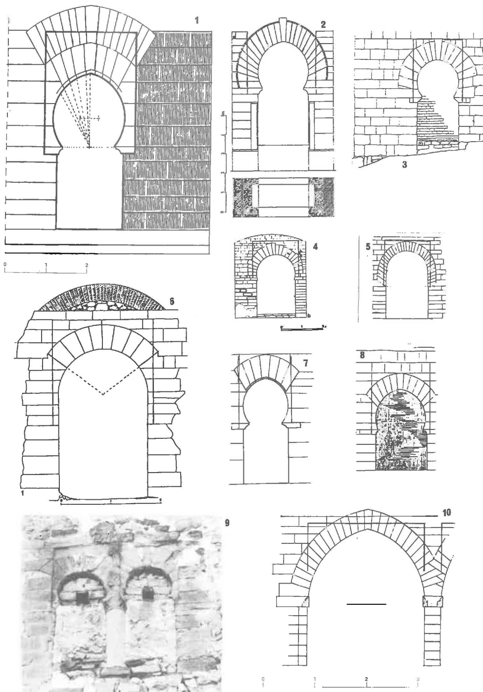
Fig.6. Arcos de puertas. Dovelas por fuera del aliz rehundido. 1, alminar de Hasn, Rabat (s. XII); 2, puerta de la Pastora. Medina Sidonia (s. XII); 3, puerta del Buey, Niebla (s. XII); 4, puerta de Mig, Denia, según Azuar (ss. XI-XII); 5, puerta del León, Alcázar de Sevilla (ss. XII-XIII); 6, puerta del Castillo de Alcaudete (s. XII); 7, arco del Alcázar cristiano, Córdoba (ss. XII-XIII); 8, puerta de Belén, Córdoba (ss.XII-XIII); 9, ventana, Castillo de Priego, Córdoba (s.s.XII-XIII); 10, de fuente callejera, Rabat
