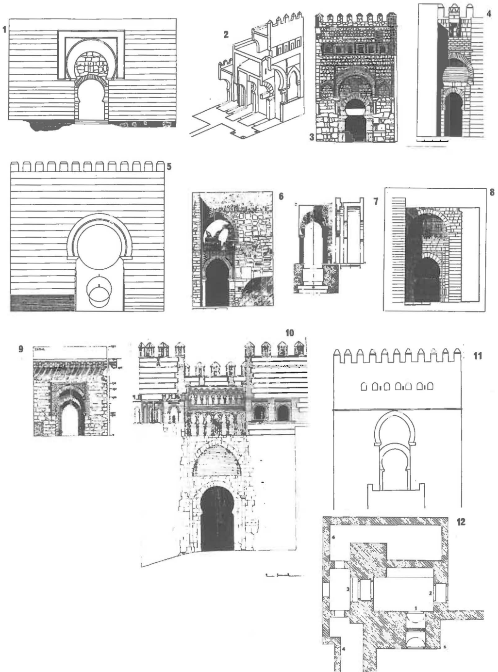
Fig. 5. Puertas con arco mayor de Buhedera: 1, Castillo de Gomar (s. X); 2-3, puerta de Bisagra Vieja, Toledo (ss. X-XI); 4, puerta de Sevilla, Carmona (ss. XII-XIII); 5, arco exterior de la puerta de Elvira, Granada (ss. XII-XIII); 1, altura de puerta de Monaita; 2, altura de puerta de las Pesas; 6, Castillo de Jimena de la Frontera, Cádiz (ss. XIII-XIV); 7, puerta de los Molinos, Ronda (s. XIII); 8, puerta del Losal, Úbeda (ss. XIV-XV); 9, puerta del Castillo de Marchena, Carmona (s. XIV); 10, puerta del Sol, Toledo (s. XIV); 11, puerta del Puente de San Martín, Toledo (s. XIV); 12, restitución de la puerta de Elvira de Granada: 1, puerta del s. XI; 3, puerta exterior con supuesta buhedera (ss. XII-XIII); 4 barbacana
