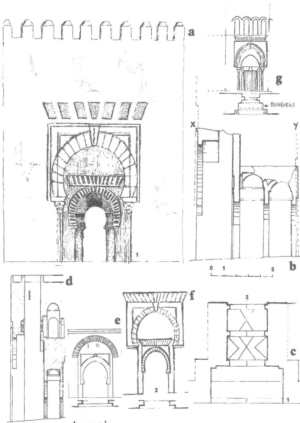
Fig. 8. Aproximación de alzado, planta y sección de Bibarramba = Orejas, de dibujos publicados por L. Torres Balbás al dibujo de Mellado publicado en 1851. A, esquema de puerta sacado del grabado de Mellado; B, sección de Bibarramba = Orejas, publicada por L. Torres Balbás. (A y B a la misma escala. En el dibujo B la "x" indica resalte exterior; la línea discontinua exterior es rasante de supuesto enchapado de la portada exterior de Mellado; la "y" indica vertical del supuesto enchapado de portada de Mellado, según nuestra propuesta segunda); C, planta de Bibarramba = Orejas, publicada por L. Torres Balbás; D, sección del inicio de la puerta de la Justicia de la Alhambra; E, portada exterior de Bib Alou de Rabat (s. XII), con arco exterior ligeramente realzado del plano del arco exterior; F, parecido aspecto de la portada de Mellado llevada a la vertical y de la sección B, según nuestra segunda propuesta; G, puerta de Ribā de Monastir (s. XI)
