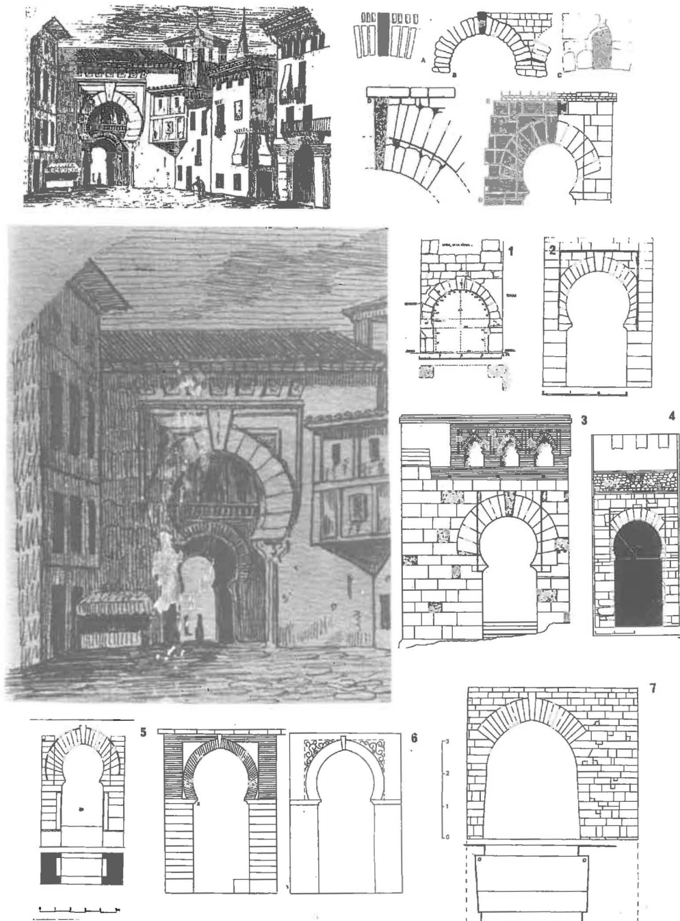
Fig. 4. Bibarrambra = puerta de las Orejas, según grabado de Mellado (1851). A, ampliación en B. puertas con dovela clave más larga; A, arco puente de Guadalajara, s. X; arco de puente romano de Hona; C, arco de puente del Acueducto de Segovia; D, puerta árabe de Maqueda (Toledo), s. X; E, puerta del Agua, Niebla, s. XII; 1, puerta de la Alcazaba de Mérida, s. IX (Félix Hernández); 2, puerta de Córdoba, Sevilla, s. XII; 3, puerta del Busey, Niebla, s. XII; 4, puerta del capitel. Alcazaba de Badajoz, s. XII; 5, puerta de la Pastora, Medina Sidonia, s. XII; 6, puerta del Castillo de Véjer de la Frontera, Cádiz, s. XII; 7, puerta del Pópulo, Cádiz, ss. XII-XIII
