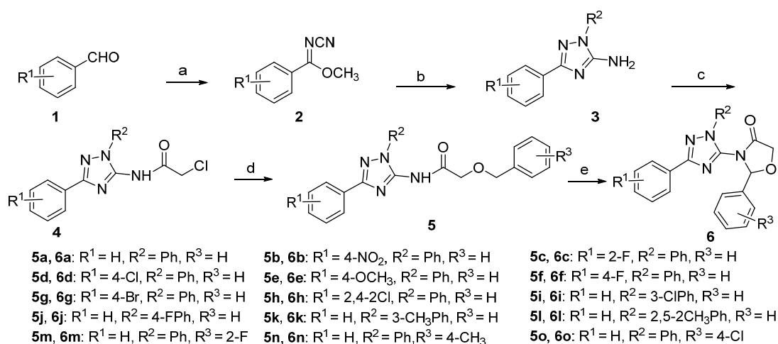
图式 1 目标化合物的合成路线
