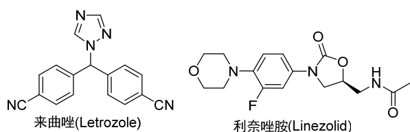
图 1 来曲唑和利奈唑胺的结构
