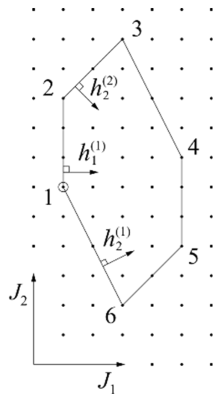
Рис. 1. Гексагональный тайл T_6
