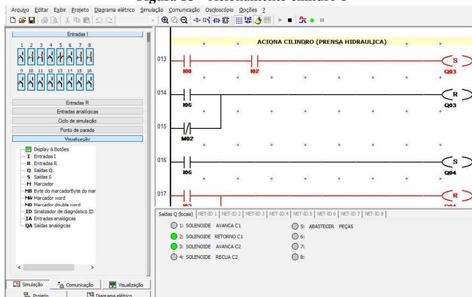
Figura 18 – Acionamento cilindro 1
