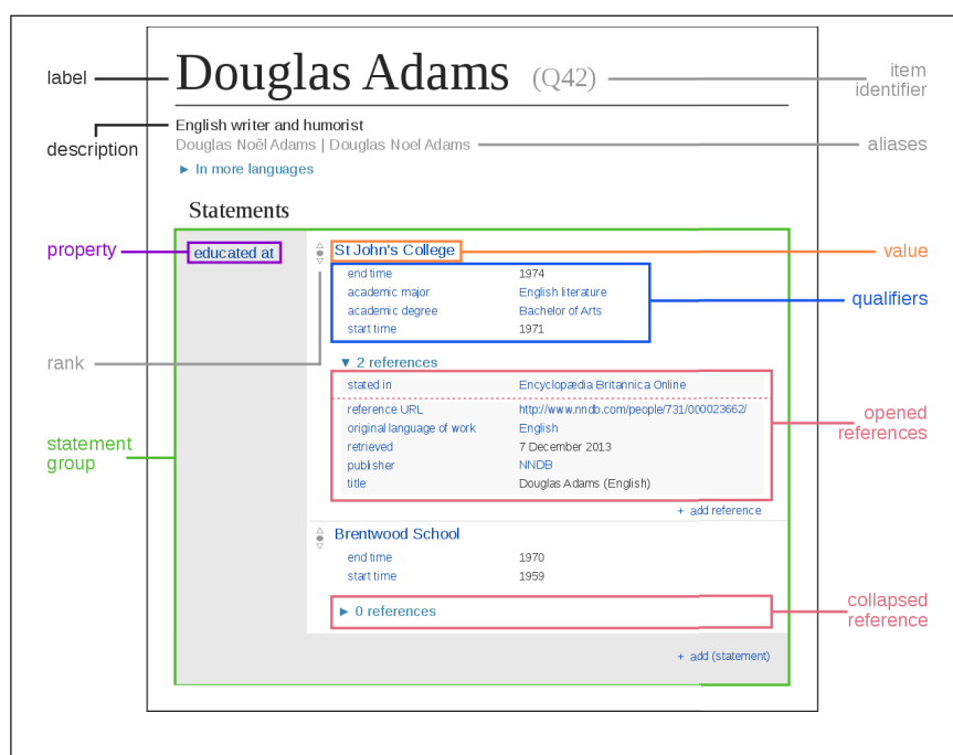
Figure 3. Datamodel in Wikidata 41
