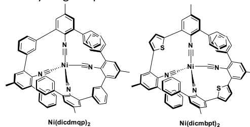
Fig. 10 Nickel isocyanide complexes.
